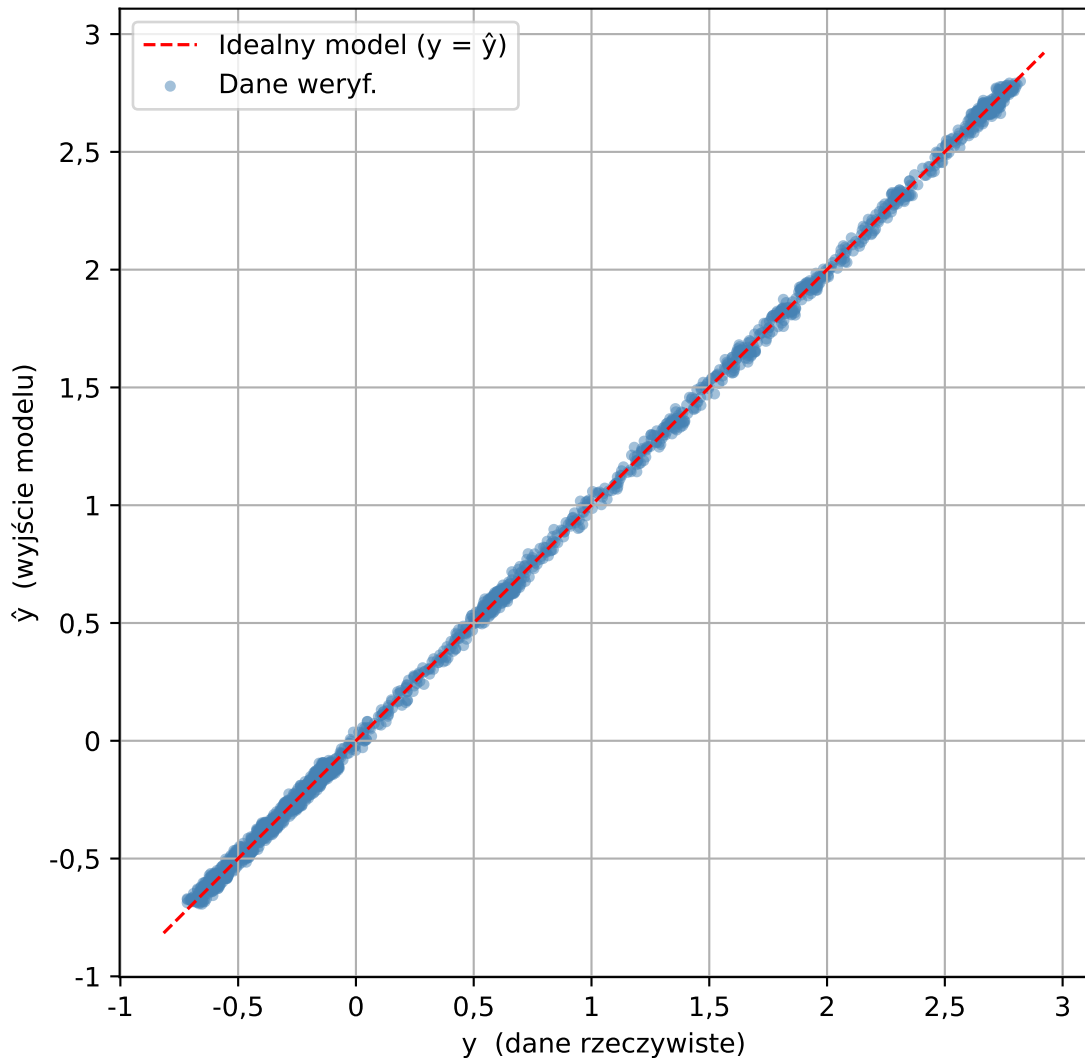
Relacja danych weryf. vs NARX( n_A=14 , \text{deg}=5 ) - bez rekurencji
