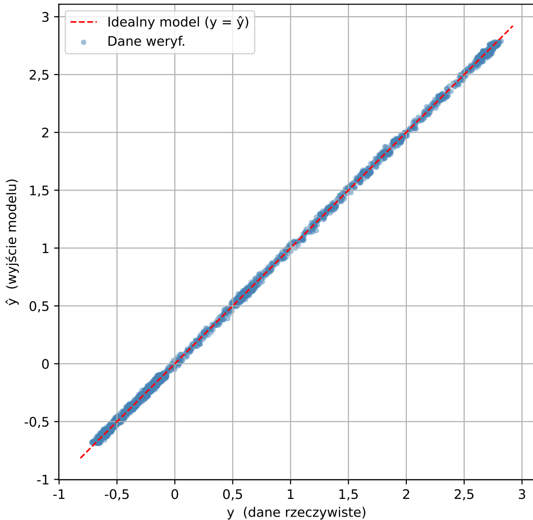
Relacja danych weryf. vs NARX( n_A=15 , \text{deg}=3 ) - bez rekurencji
