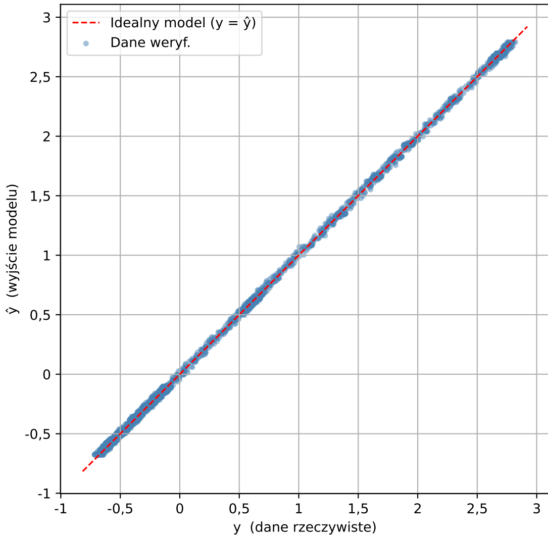
Relacja danych weryf. vs NARX(nA=15, deg=4) - z rekurencją
