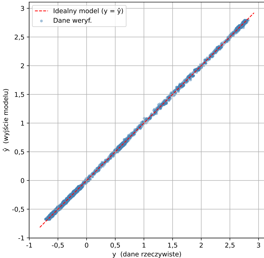
Relacja danych weryf. vs NARX(nA=15, deg=5) - z rekurencją
