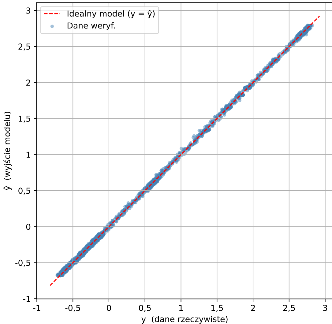
Relacja danych weryf. vs NARX(nA=15, deg=6) - z rekurencją
