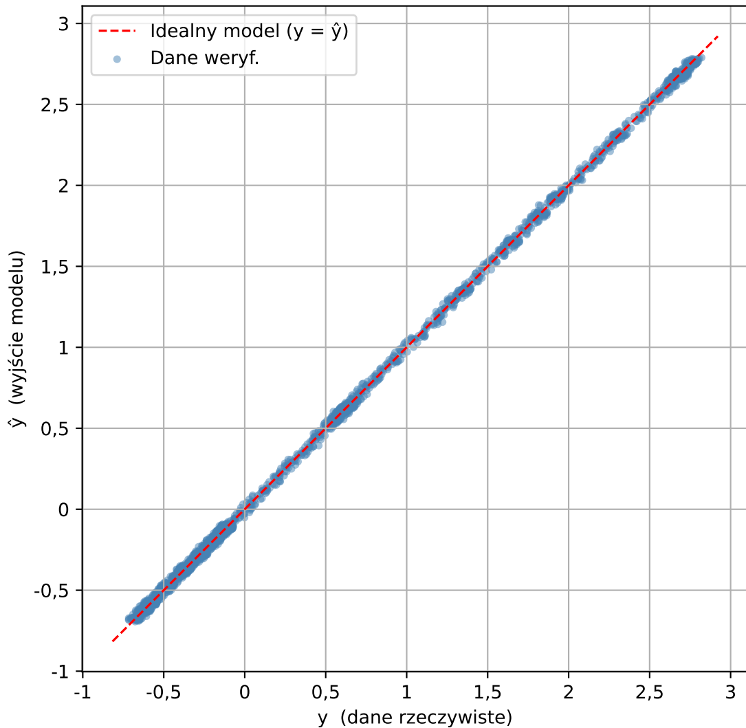
Relacja danych weryf. vs NARX( n_A=16 , \text{deg}=3 ) - bez rekurencji
