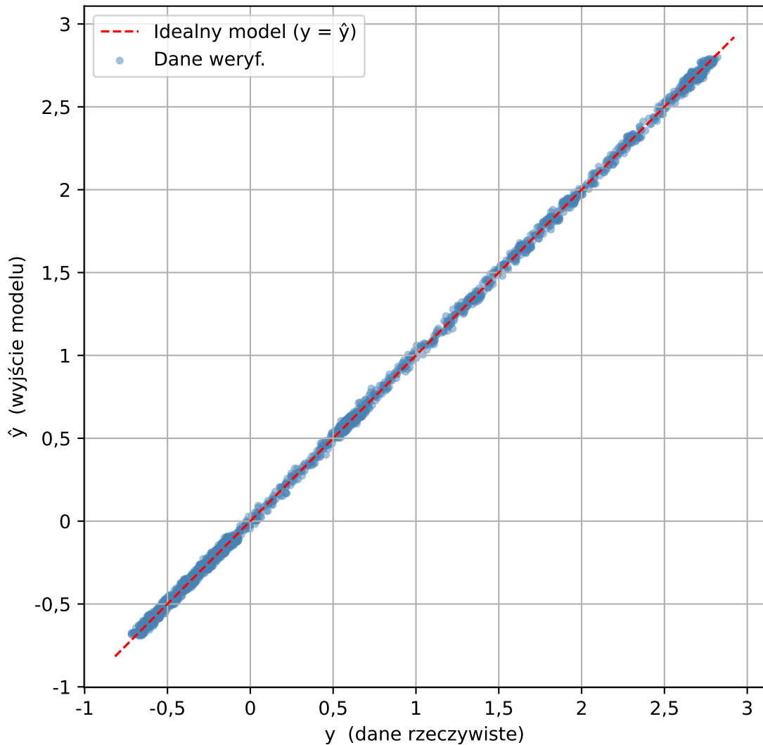
Relacja danych weryf. vs NARX( n_A=16 , \text{deg}=4 ) - bez rekurencji
