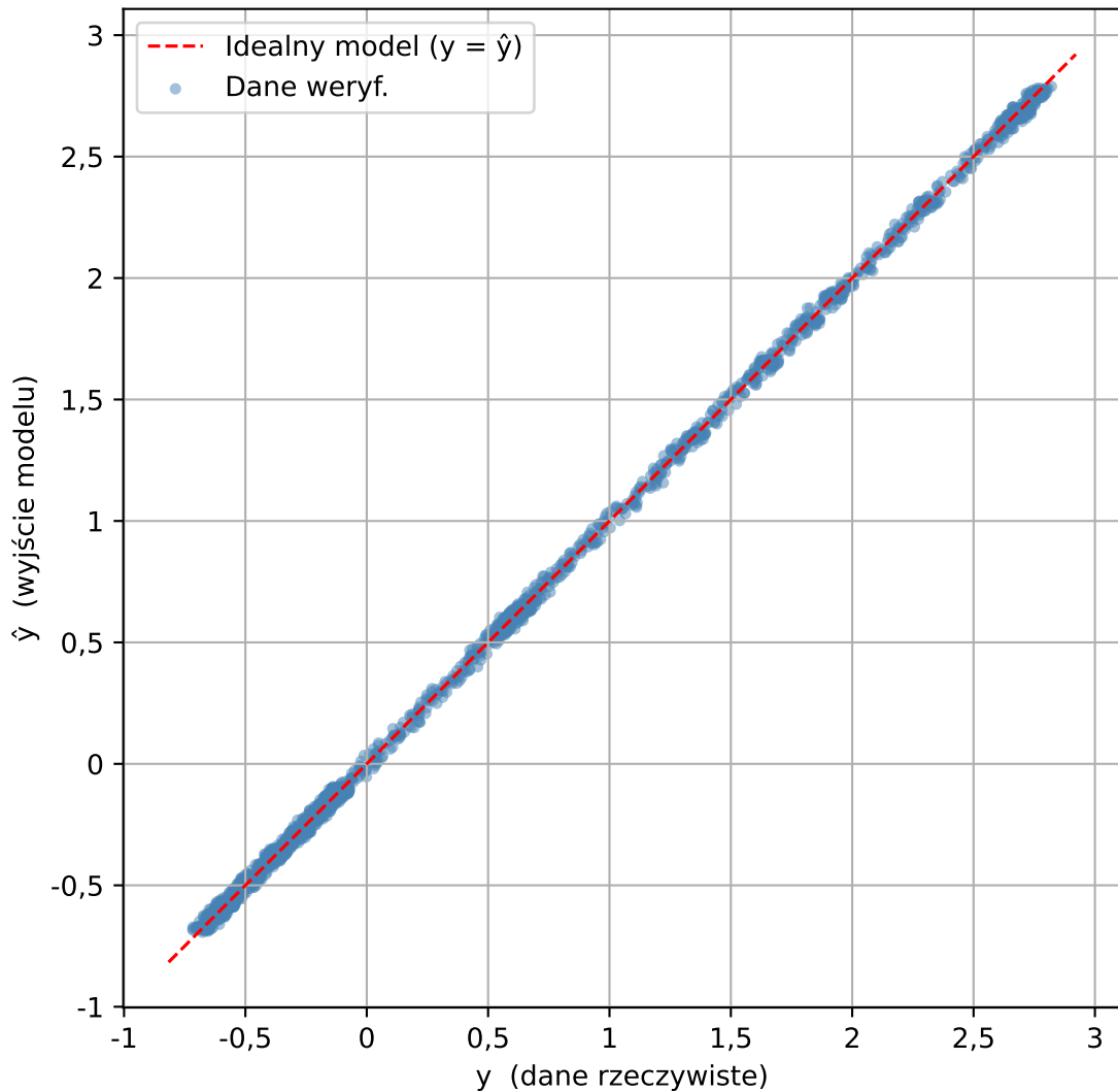
Relacja danych weryf. vs NARX( n_A=17 , \text{deg}=3 ) - bez rekurencji
