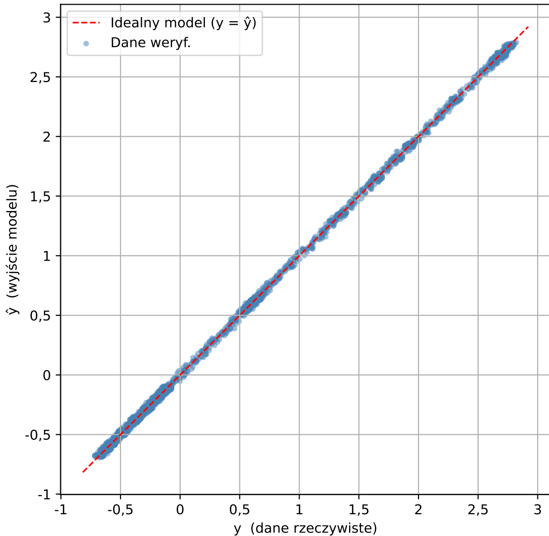
Relacja danych weryf. vs NARX( n_A=18 , \text{deg}=3 ) - bez rekurencji
