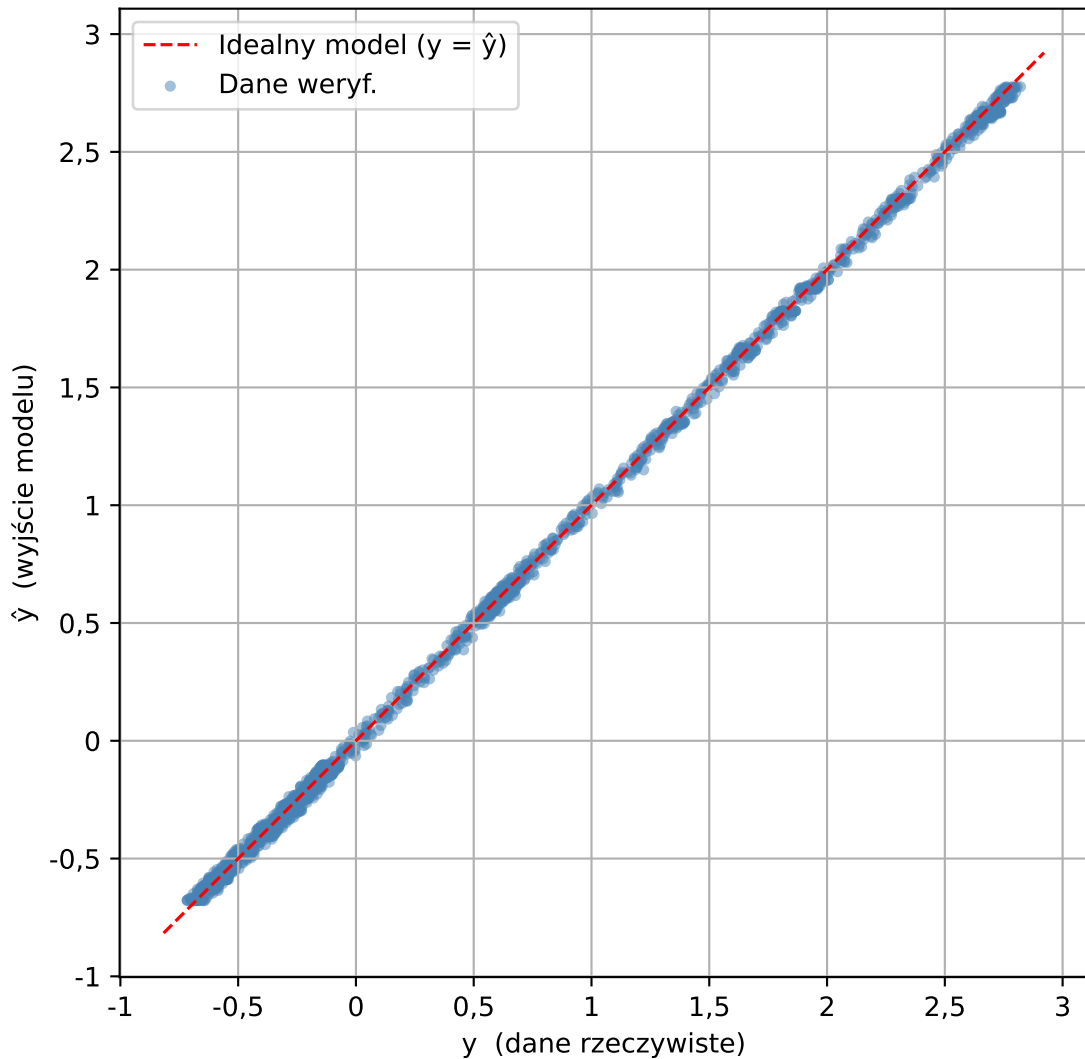
Relacja danych weryf. vs NARX(nA=18, deg=3) - z rekurencją
