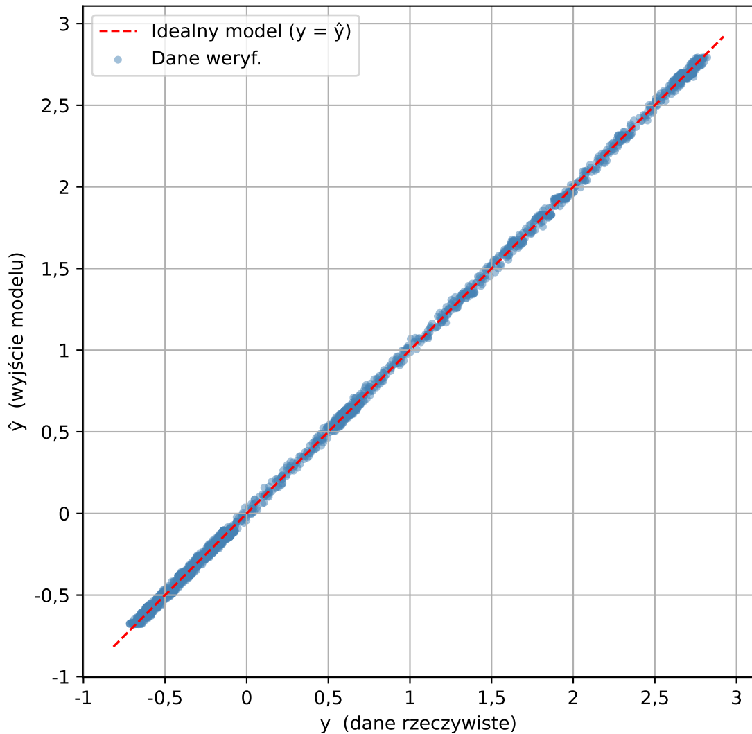
Relacja danych weryf. vs NARX(nA=18, deg=4) - z rekurencją
