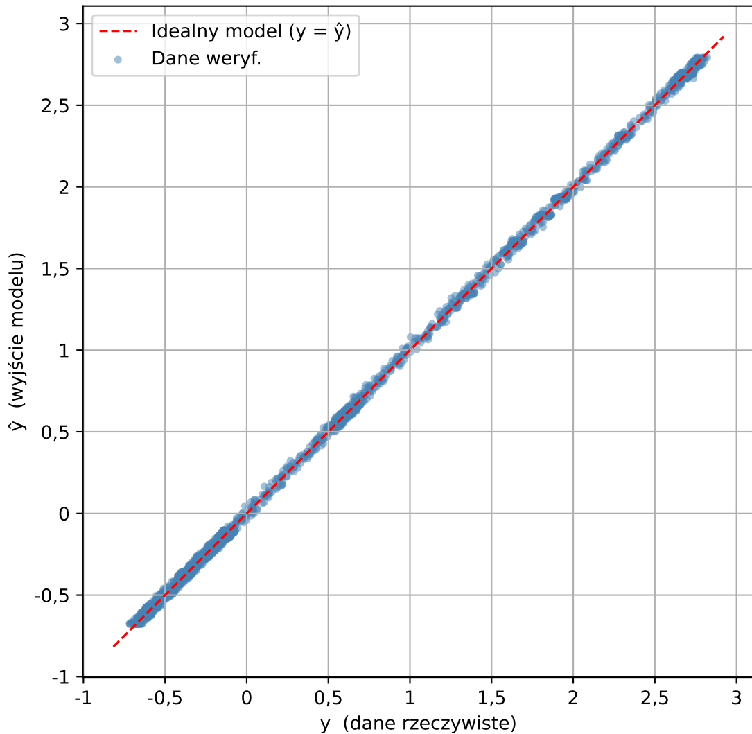
Relacja danych weryf. vs NARX(nA=18, deg=5) - z rekurencją
