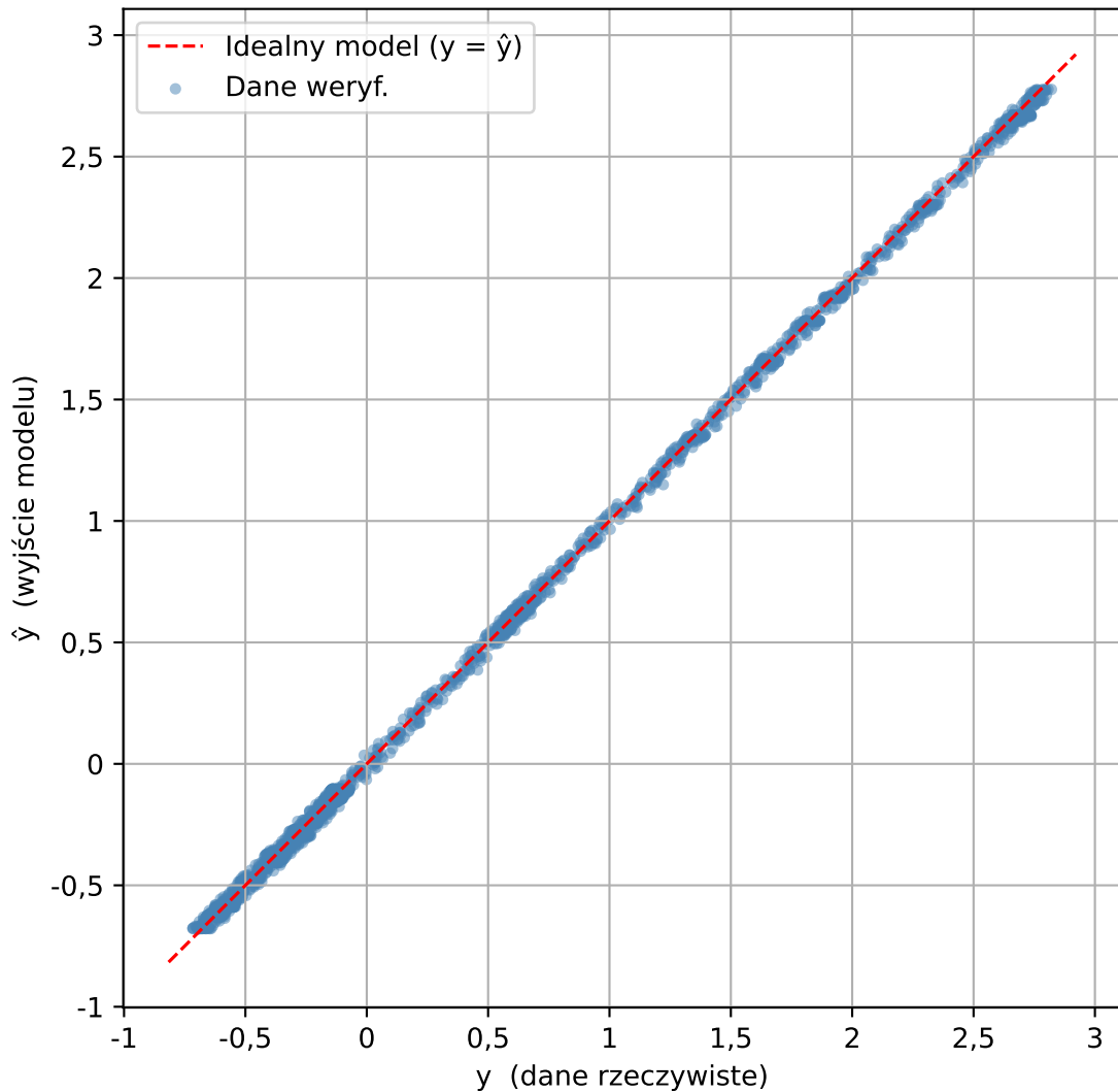
Relacja danych weryf. vs NARX(nA=19, deg=3) - z rekurencją
