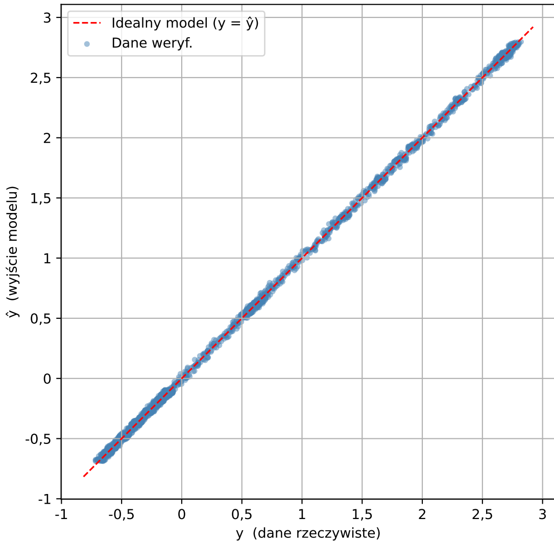
Relacja danych weryf. vs NARX( n_A=19 , \text{deg}=4 ) - bez rekurencji
