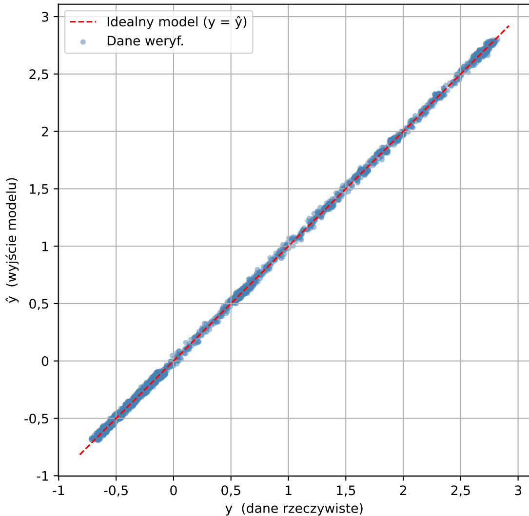
Relacja danych weryf. vs NARX( n_A=19 , \text{deg}=5 ) - bez rekurencji
