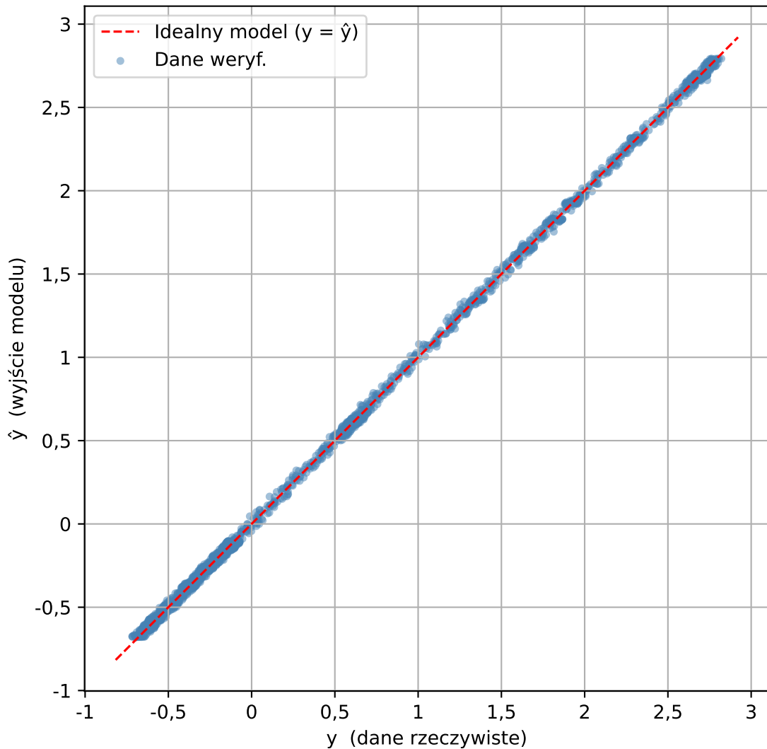
Relacja danych weryf. vs NARX(nA=19, deg=5) - z rekurencją
