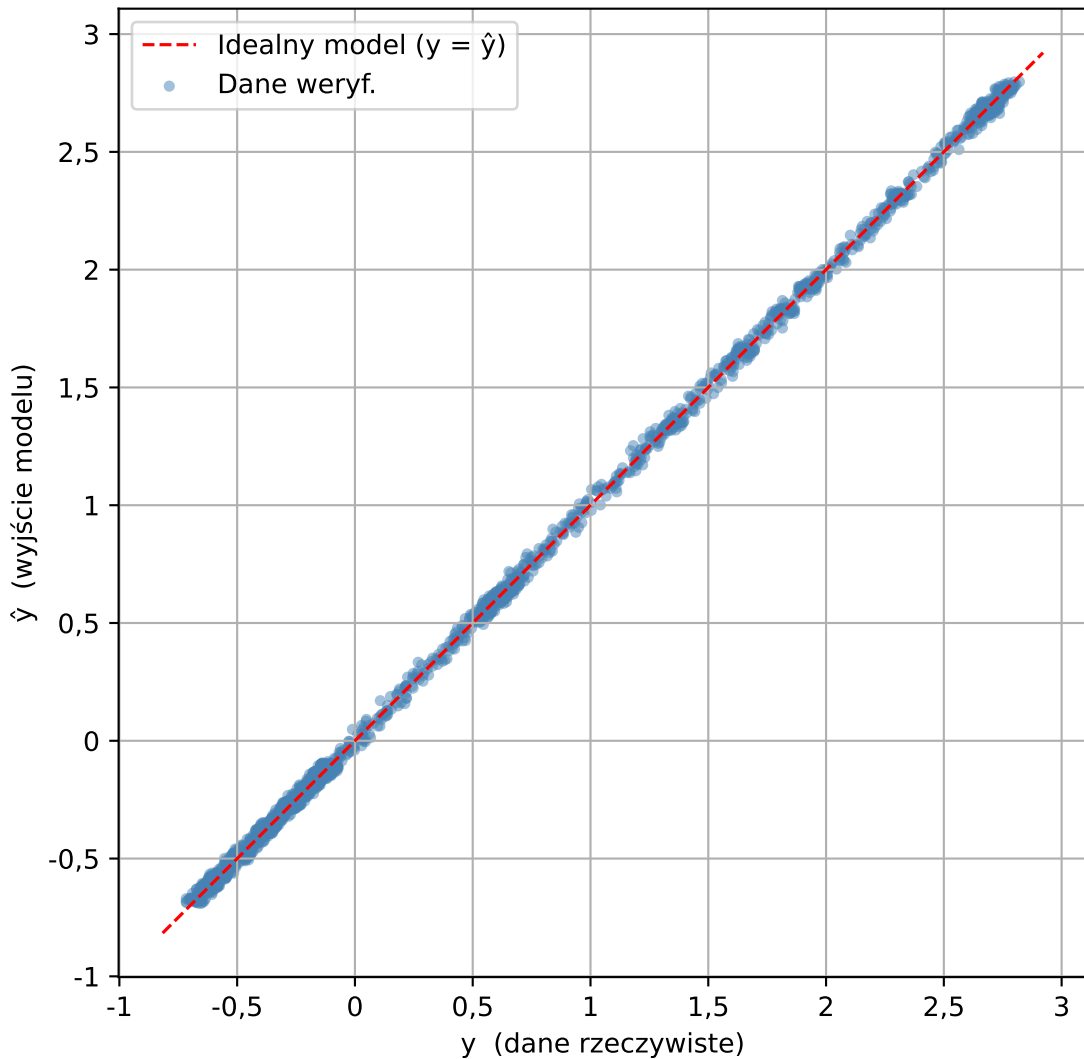
Relacja danych weryf. vs NARX( n_A=19 , \text{deg}=6 ) - bez rekurencji
