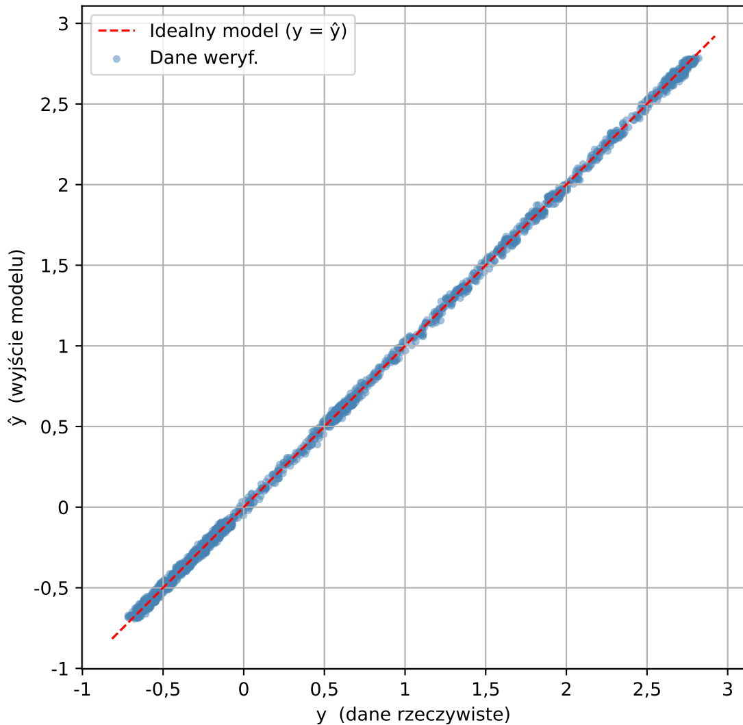
Relacja danych weryf. vs NARX( n_A=20 , \text{deg}=3 ) - bez rekurencji
