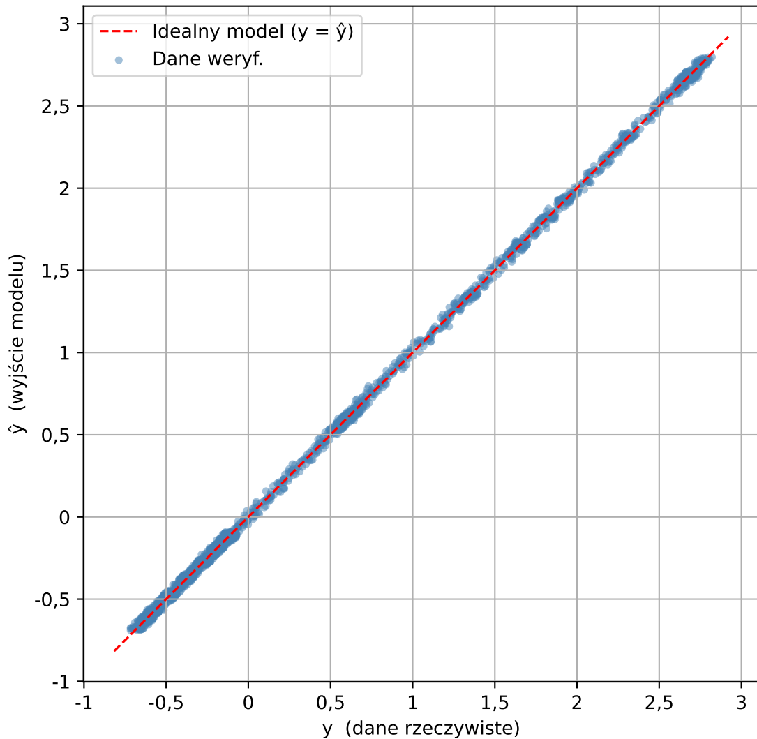
Relacja danych weryf. vs NARX( n_A=20 , \text{deg}=4 ) - bez rekurencji
