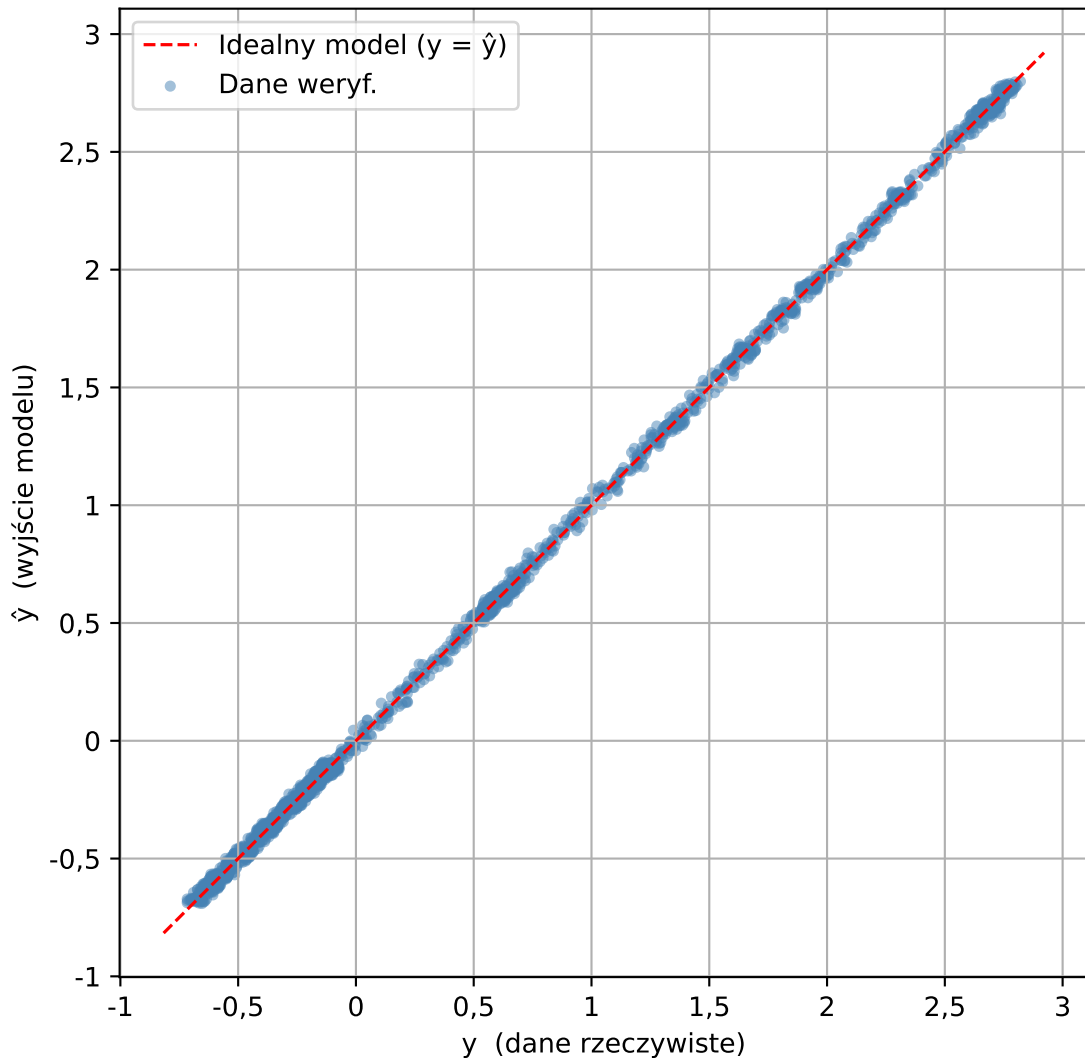
Relacja danych weryf. vs NARX( n_A=20 , \text{deg}=5 ) - bez rekurencji
