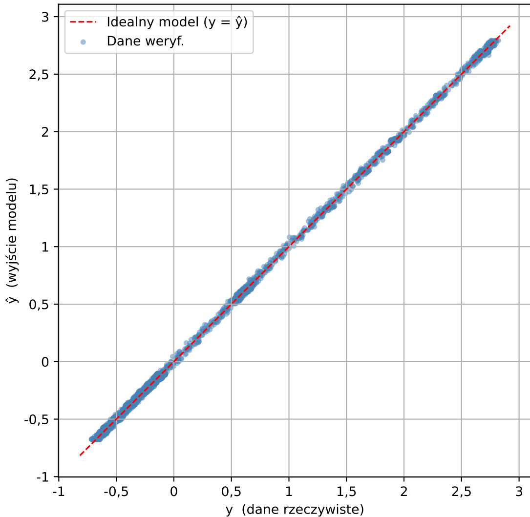
Relacja danych weryf. vs NARX(nA=20, deg=5) - z rekurencją
