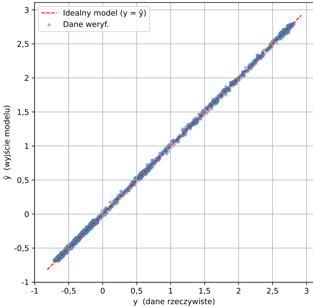
Relacja danych weryf. vs NARX( n_A=20 , \text{deg}=6 ) - bez rekurencji
