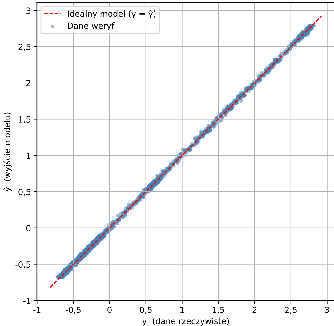
Relacja danych weryf. vs NARX(nA=20, deg=6) - z rekurencją
