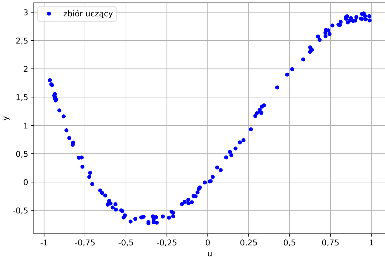
Charakterystyka statyczna - zbiór uczący (60 %)
