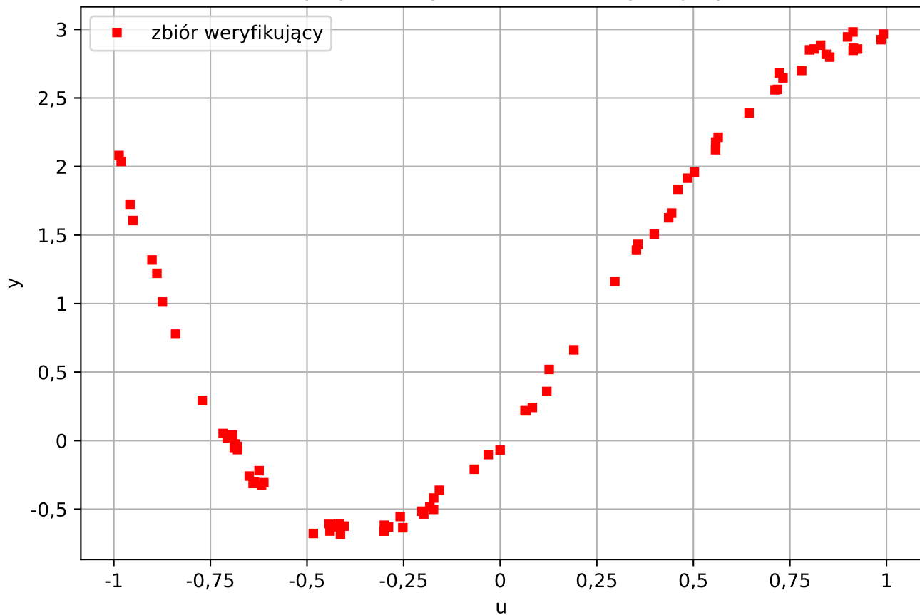
Charakterystyka statyczna - zbiór weryfikujący (40 %)
