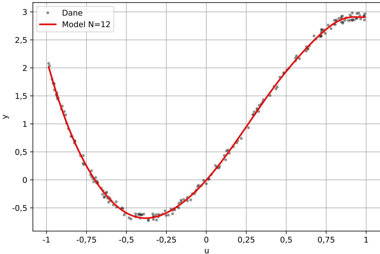
Charakterystyka statyczna - model wielomianowy N=12
