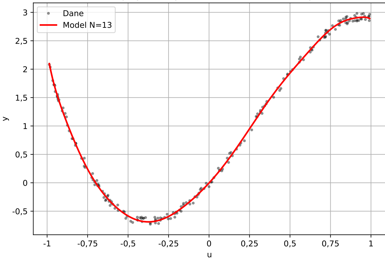
Charakterystyka statyczna - model wielomianowy N=13
