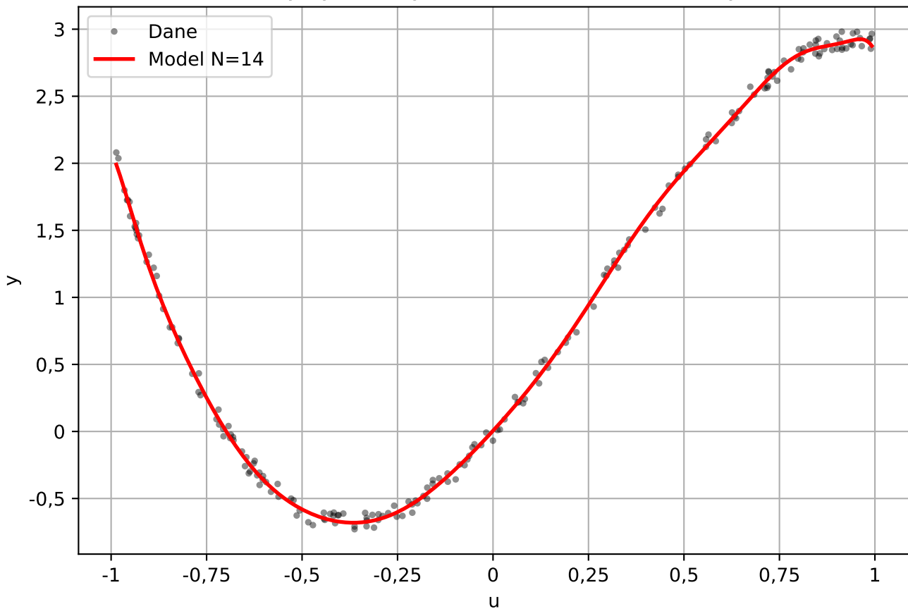
Charakterystyka statyczna - model wielomianowy N=14
