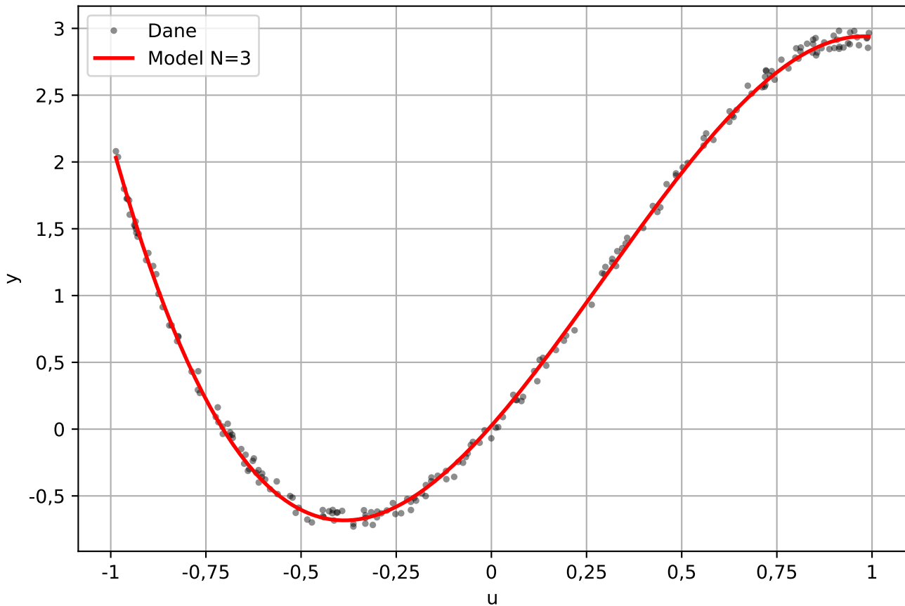
Charakterystyka statyczna - model wielomianowy N=3
