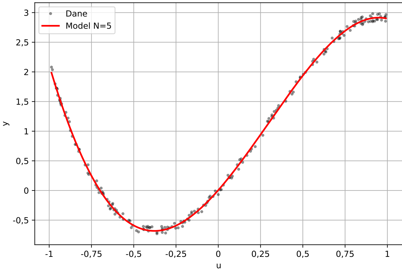
Charakterystyka statyczna - model wielomianowy N=5
