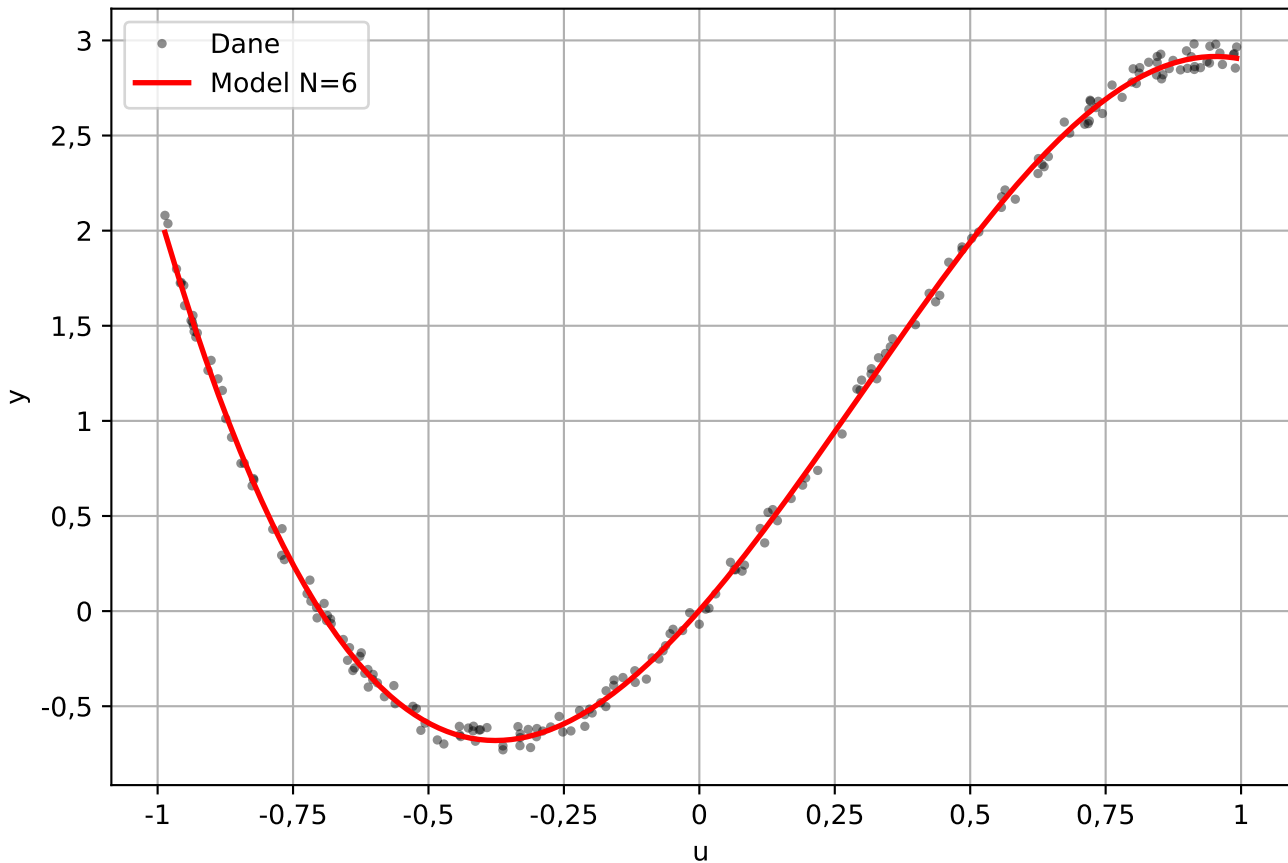
Charakterystyka statyczna - model wielomianowy N=6
