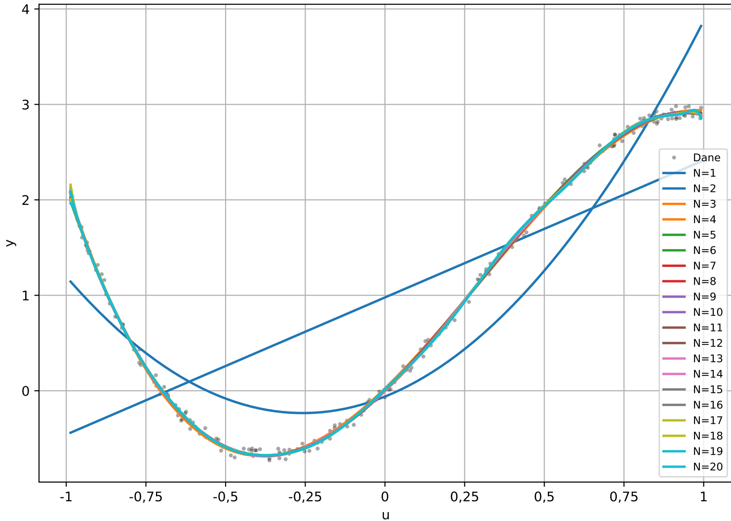
Charakterystyki statyczne - wszystkie modele wielomianowe
