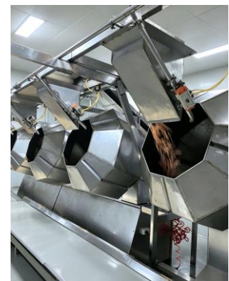
(Lồng quay phun gia vị tự động hình bát giác)
