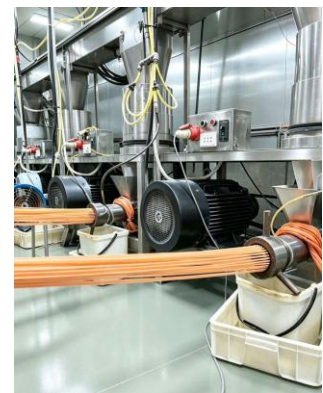
(Cụm máy ép đùn trực vít sinh nhiệt nở phòng trực tiếp)
