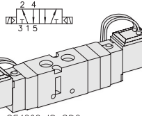
SF4303-IP-SD2-*** 2 4 3 1 5
