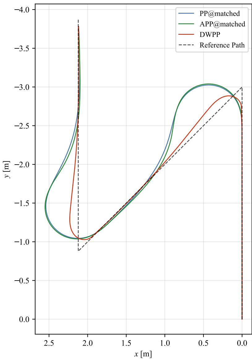
PathC
