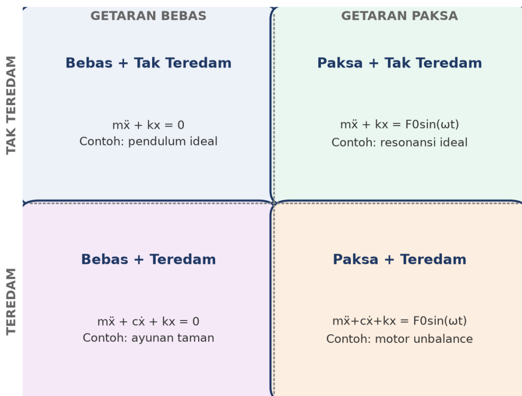
Gambar 3. Klasifikasi getaran berdasarkan dua dimensi: ada/tidak gaya eksitasi (bebas vs paksa) dan ada/tidak elemen redaman (tak teredam vs teredam).
