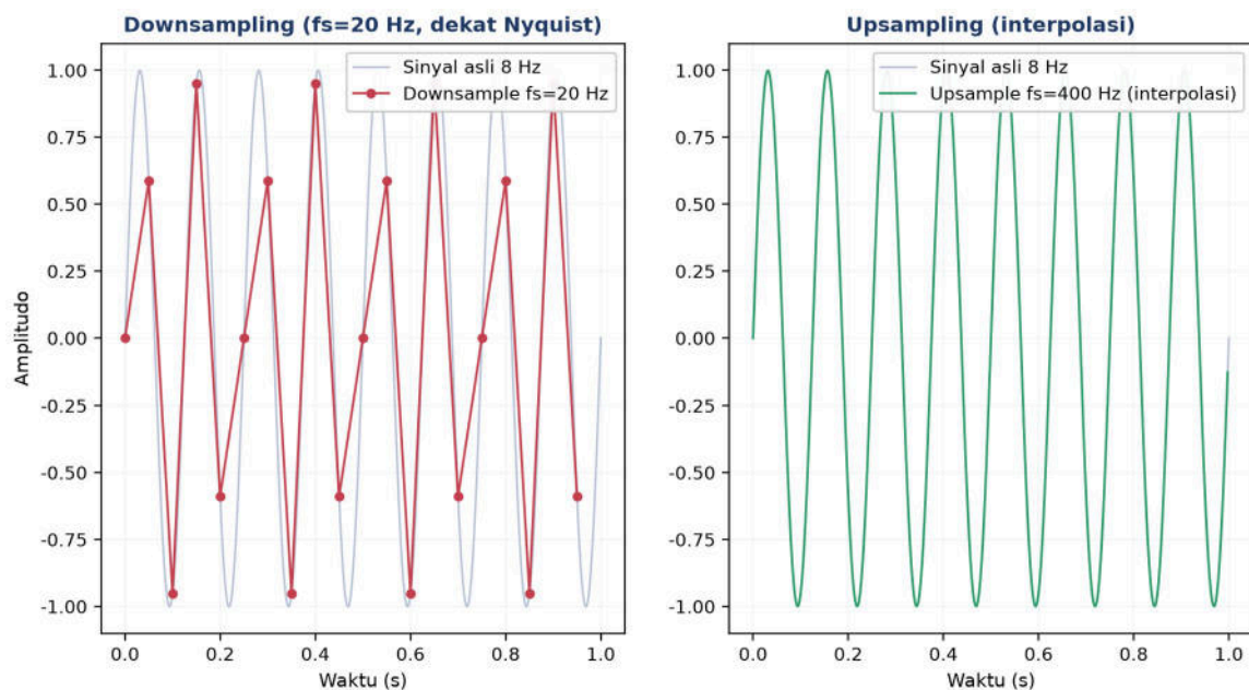
Gambar 6 Ilustrasi downsampling ( fs=20\text{ Hz} , dekat batas Nyquist) dan upsampling via interpolasi pada sinyal 8 Hz
