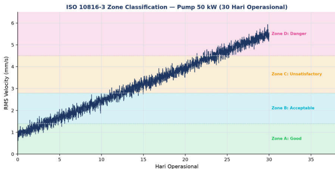
Gambar 2. Simulasi streaming RMS velocity pompa 50kW selama 30 hari operasional, dengan awal zona ISO10816-3 A-D sinyal berdegradasi dari zona A menuju D
