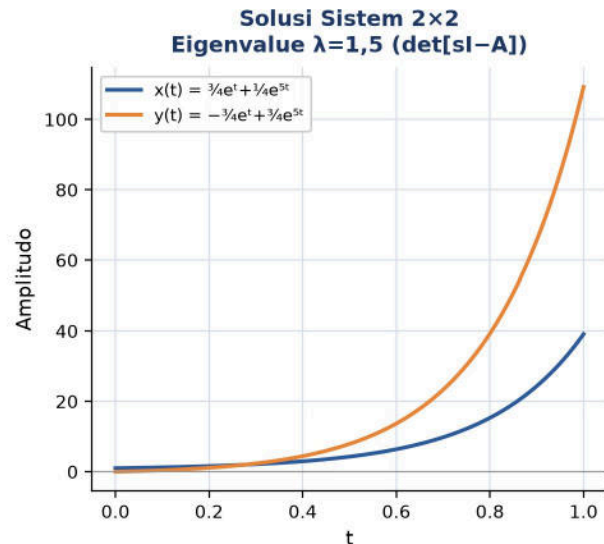
Gambar 7. Signal-flow sistem PD coupled x' = 2x + y, y' = 3x + 4y (kiri) dan solusi x(t), y(t) hasil solve matriks dengan eigenvalue \lambda = 1, 5 (kanan).
