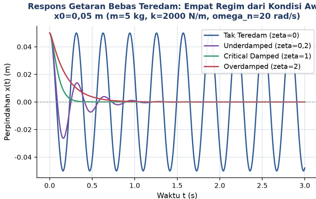
Gambar 3. Respons getaran bebas teredam untuk empat regim ( \zeta=0; 0,2; 1; 2 ) dari kondisi awal yang sama, dihitung dengan integrasi Runge-Kutta orde 4.
