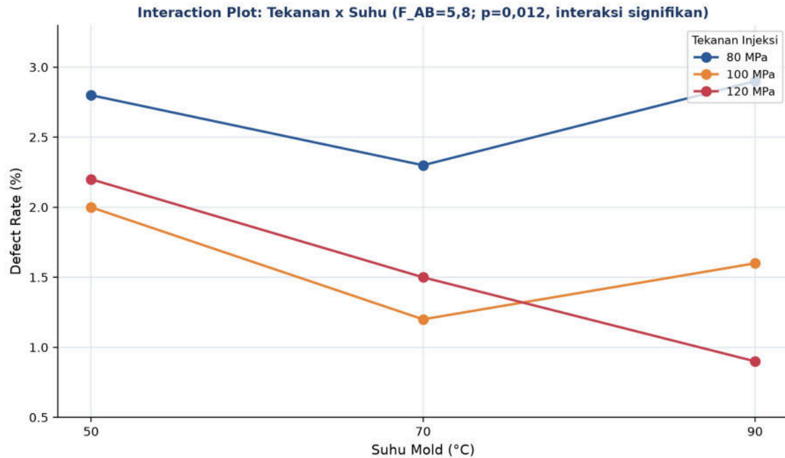
Gambar 5. Interadion plot tekanan injeksi x suhu mold: garis tidak paralel menandakan interaksi signifikan; kombinasi optimal 120 MPa & 90°C (defect terendah).
