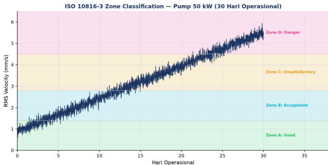
Gambar 2. Simulasi streaming RMS velocity pompa 50kW selama 30 hari operasional, dengan overlay zona ISO 10816-3 A-D sinyal berdegradasi dari zona A menuju ke D
