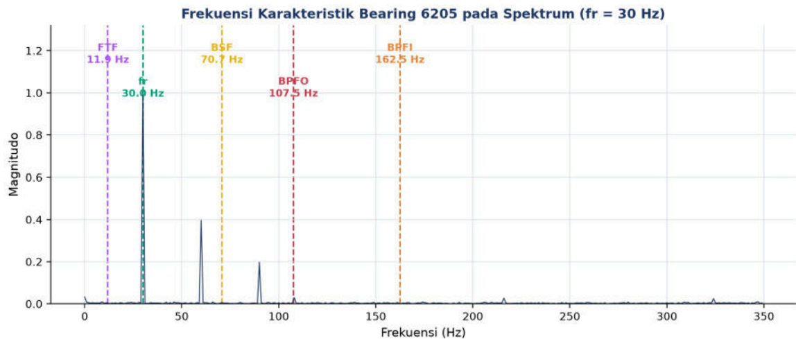
Gambar 5 Spektrum sinyal bearing 6205 dengan overlay garis frekuensi karakteristik FTF, fr, BSF, BPFO, dan BRFI ( fr=30\text{ Hz} ).
