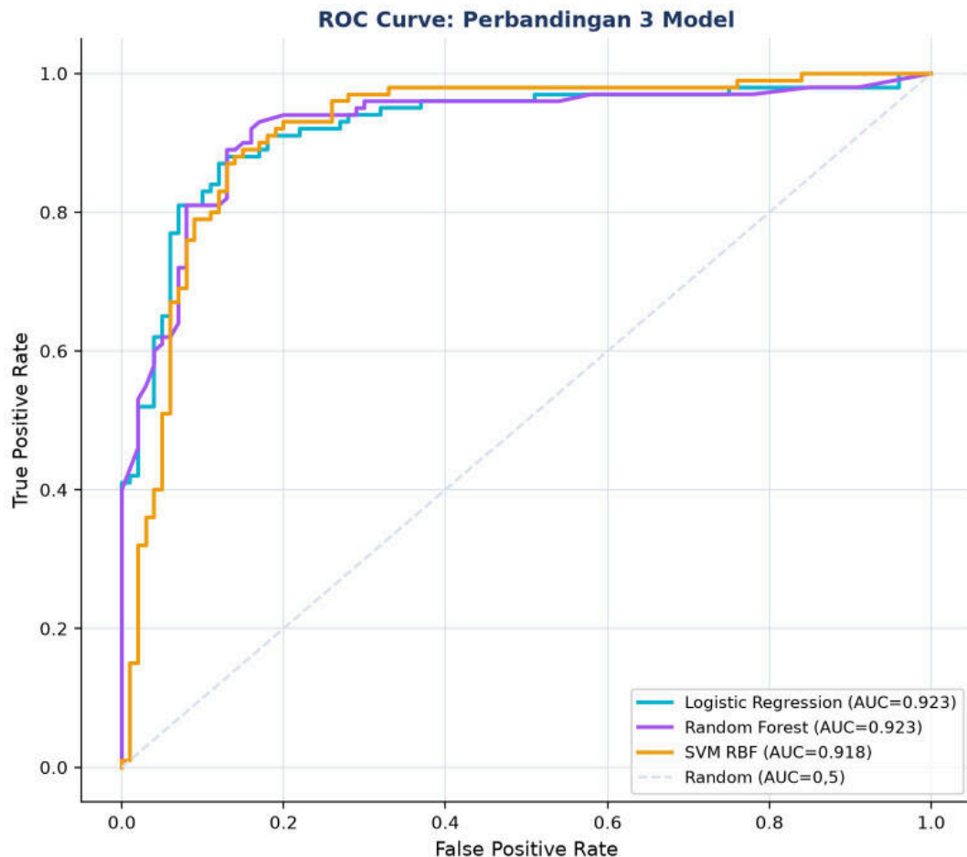
Gambar 4. Kurva ROC tiga model (Logistic Regression, Random Forest, SVM RBF) pada dataset dengan overlap kelas lebih realistis; AUC mengukur kemampuan model me-rankir sampel positif di atas negatif, independen dari threshold
