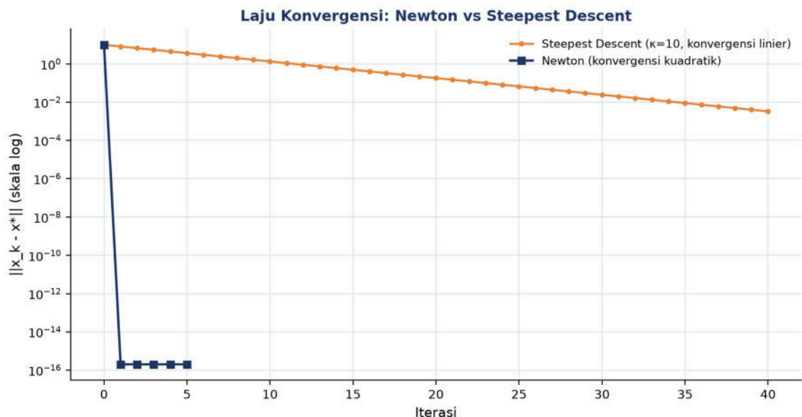
Gambar 3 Perbandingan laju konvergensi Newton (kuadratik) vs Steepest Descent (linier, condition number \kappa \neq 1 ) pada fungsi kuadratik
