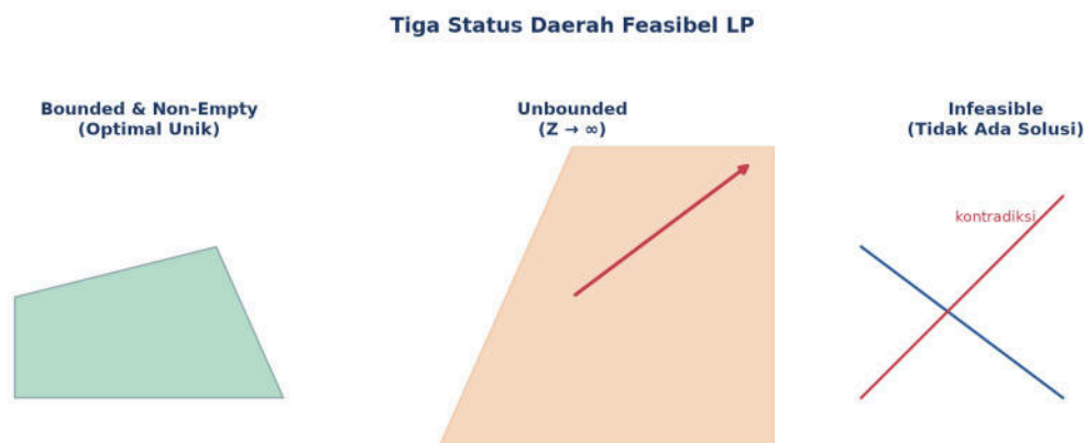
Gambar 3 | lustrasi visual tiga status utama daerah feasible: bounded & non-empty unbounded, dan infeasible.
