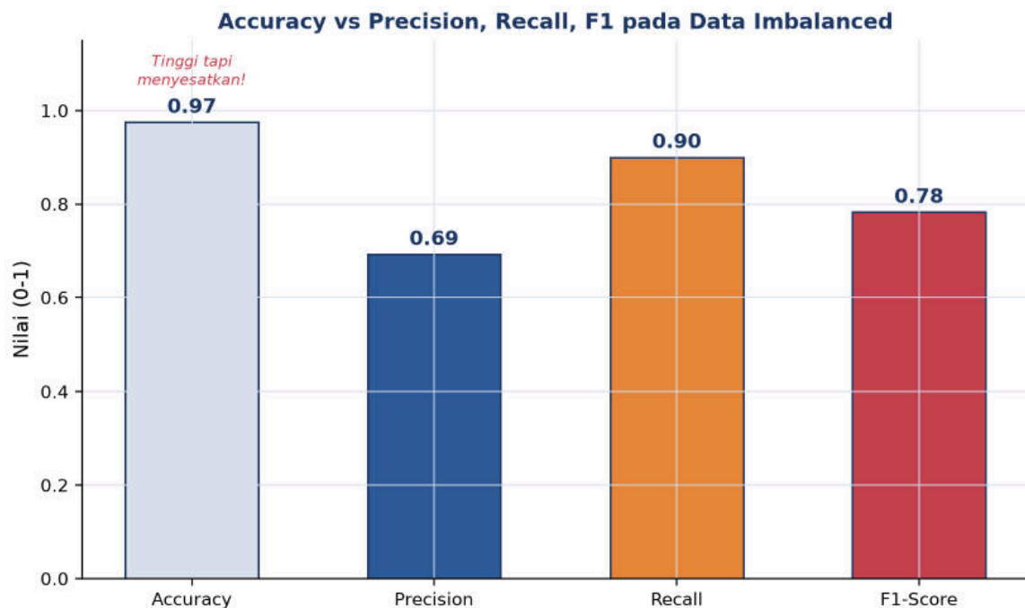
Gambar 5. Accuracy (0, 975) tampak sangat tinggi tetapi menyesatkan pada data imbalanced; precision (0, 69), recall (0, 90), dan F1 (0, 78) memberi gambaran lebih jujur tentang kinerja a model.
