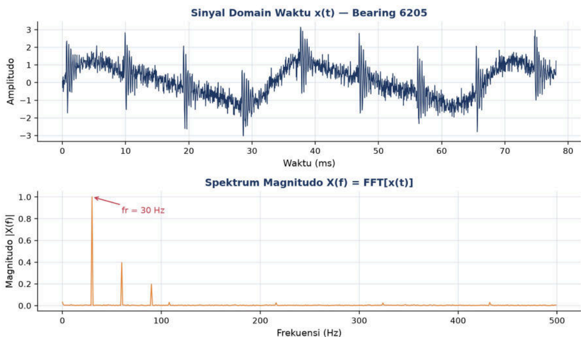
Gambar 2 Sinyal domain waktu x(t) bearing 6205 (atas) dan spektrum magnitudo hasil FFT X(f) (bawah), dengan peak fr=30\text{Hz} .
