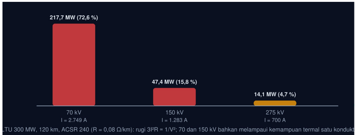
Gambar 2 — Rugi daya terhadap tingkat tegangan untuk daya dan konduktor yang sama. PLTU 300 MW sejauh 120 km dengan ACSR 240: pada 70 dan 150 kV rugi melampaui sepersepuluh daya dan arusnya melampaui kemampuan termal konduktor; 275 kV memberi rugi 4,7 % dan 500 kV 1,4 %.
