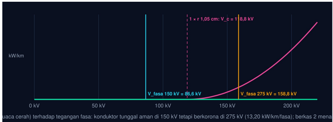
Gambar 6 — Tegangan kritis korona dan rugi korona: konduktor tunggal vs berkas. Konduktor tunggal r = 1,05 cm berkorona di atas 119 kV fasa: aman pada 150 kV, tetapi pada 275 kV membuang 13,2 kW/km/fasa. Berkas dua sub-konduktor menaikkan tegangan kritis ke 673 kV.
