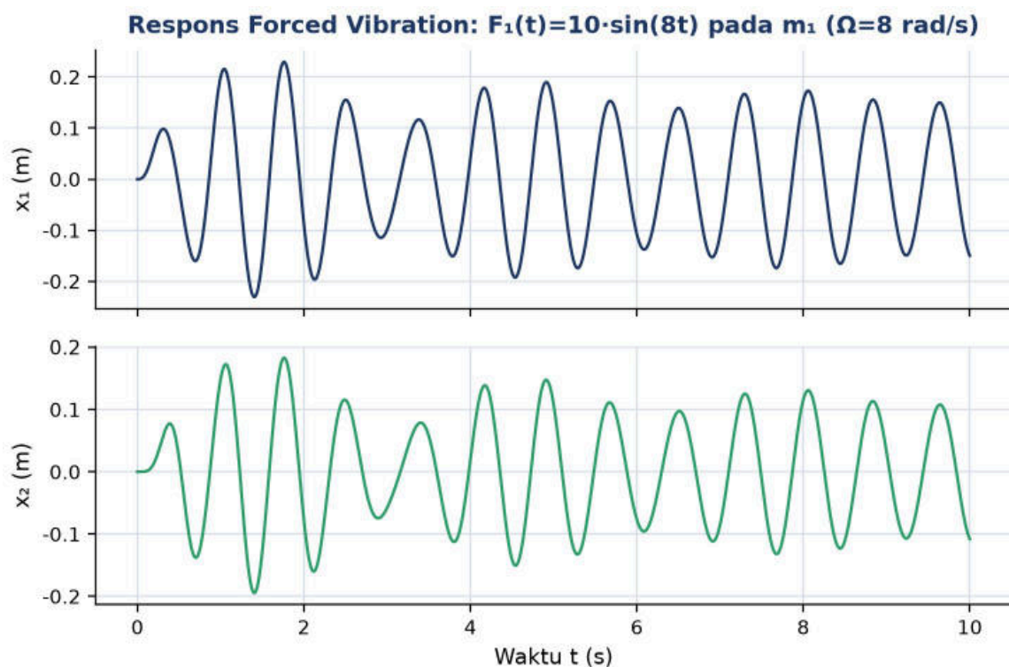
Gambar 7. Respons forced vibration sistem referensi 2-DoF hasil solve_ivp: gaya harmonik F_1(t)=10\cdot\sin(8t) diterapkan pada m_1 , respons oleh kedua massa akibat kopling pegas k_2 .
