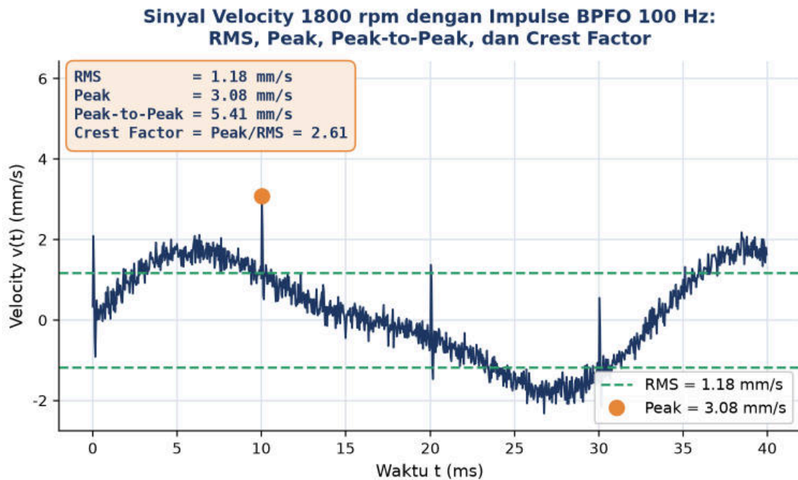
Gambar 2. Sinyal velocity 1800 rpm dengan impulse train BPFO 100 Hz garis putus-putus menandai pita RMS, titik oranye menandai Peak, dan kotak keterangan merangkum keempat nilai (RMS, Peak, Peak-to-Peak, Crest Factor).
