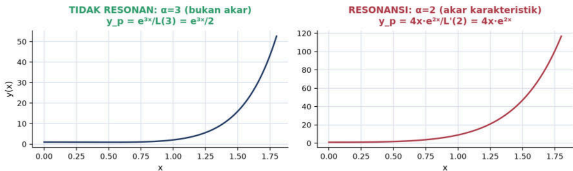
Gambar 5 Perbandingan solusi total y(x) untuk L(D)=D^2-3D+2 (akar 1, 2) dengan y(0)=1 , y'(0)=0 : kasus tidak resonan ( \alpha=3 ) tumbuh murni eksponensial, sedangkan kasus resonansi ( \alpha=2 ) mendapat faktor tambahan x yang membuatnya tumbuh lebih cepat.
