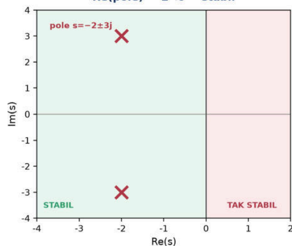
Gambar 4. Transfer function sebagai blok sistem U(s) \rightarrow H(s) \rightarrow Y(s) untuk sirkuit RLC seri (kiri) dan pole-zero plot yang menunjukkan pole s = -2 \pm 3j pada region stabil (kanan).
