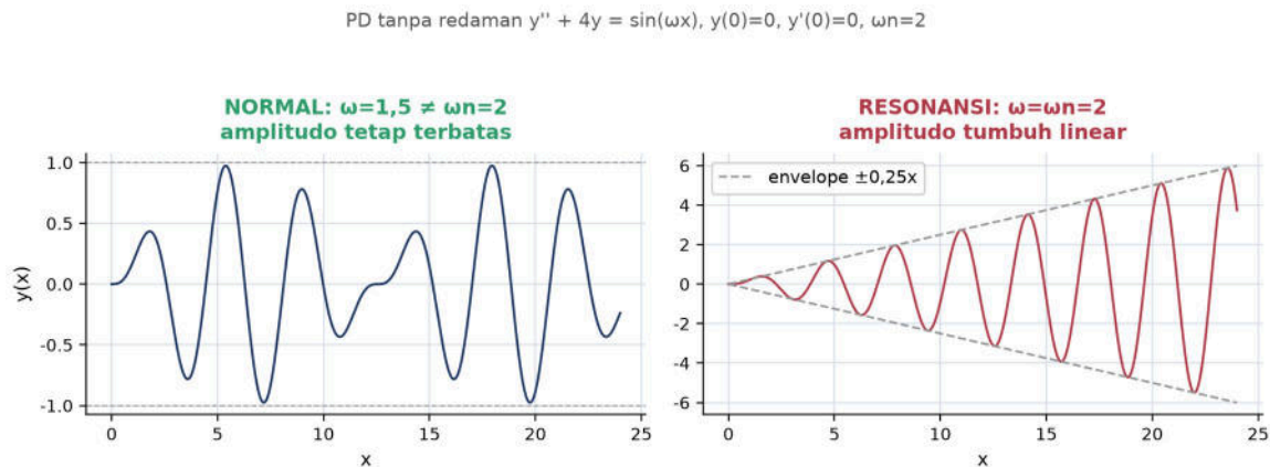
Gambar 4 Perbandingan sol usi PD tanpa redaman y'' + 4y = \sin(\omega) : panel kiri ( \omega=1,5 \neq \omega_n=2 ) amplitudo tetap terbatas; panel kanan ( \omega=2 , resonansi) amplitudo tumbuh linear dengan selubung \pm 0,25x .
