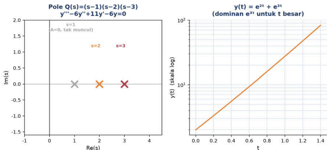
Gambar 6. Pole PD orde 3 y'''-6y''+11y'-6y=0 di s=1,2,3 (kiri) dan kurva pertumbuhan y(t)=e^{2t}+e^{3t} dalam skala log (kanan); koefisien akar s=1 kebetulan nol sehingga tak muncul di solusi akhir.
