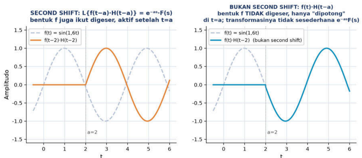
Gambar 4. Perbandingan Second Shift sejati f(t-a) \cdot H(t-a) (panel kiri, bentuk f fungsi ikut digeser) dengan bentuk yang keliru f(t) \cdot H(t-a) (panel kanan, bentuk f fungsi tidak digeser, hanya dipotong pada t=a ).
