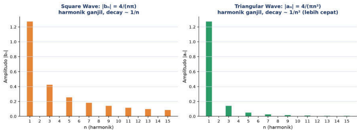
Gambar 2 Spektrum amplitudo square wave (decay \sim 1/n , harmonik ganjil) dibandingkan triangular wave (decay \sim 1/n^2 , harmonik ganjil), menunj ukkan laj u peluruhan yang j auh lebih cepat pada sinyal yang lebih halus.
