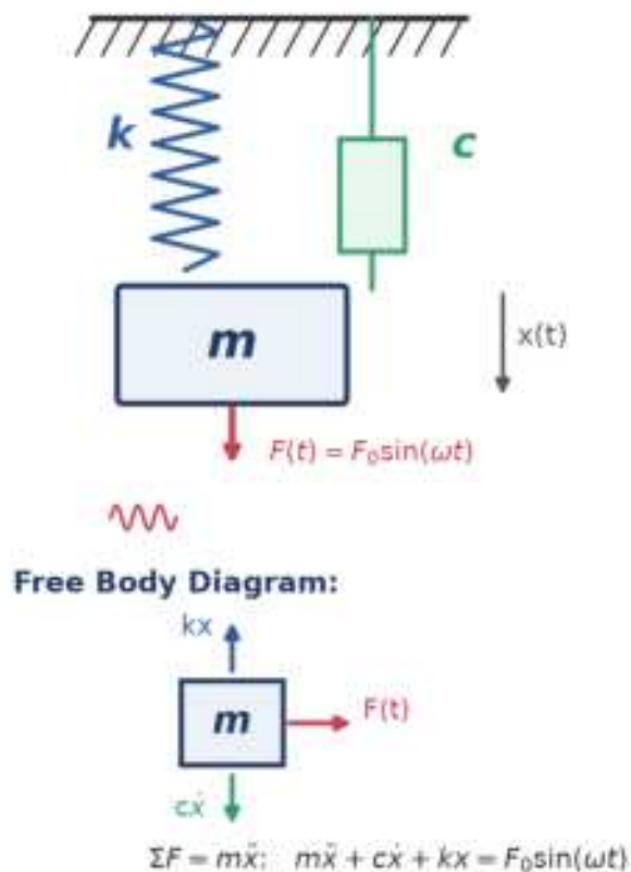
Gambar 2. Sistem getaran paksa 1-DoF (massa-pegas-peredam) dengan gaya eksitasi harmonik F(t) , beserta free body diagram gaya-gayanya.
