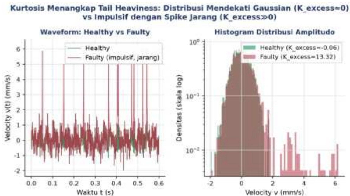
Gambar 4. Histogram distribusi amplitudo (skala log): sinyal mendekati Gaussian (excess kurtosis kira-kira nol) versus sinyal dengan spike jarang beramplitudo besar (excess kurtosis jauh di atas nol, ekor distribusi memanjang).
