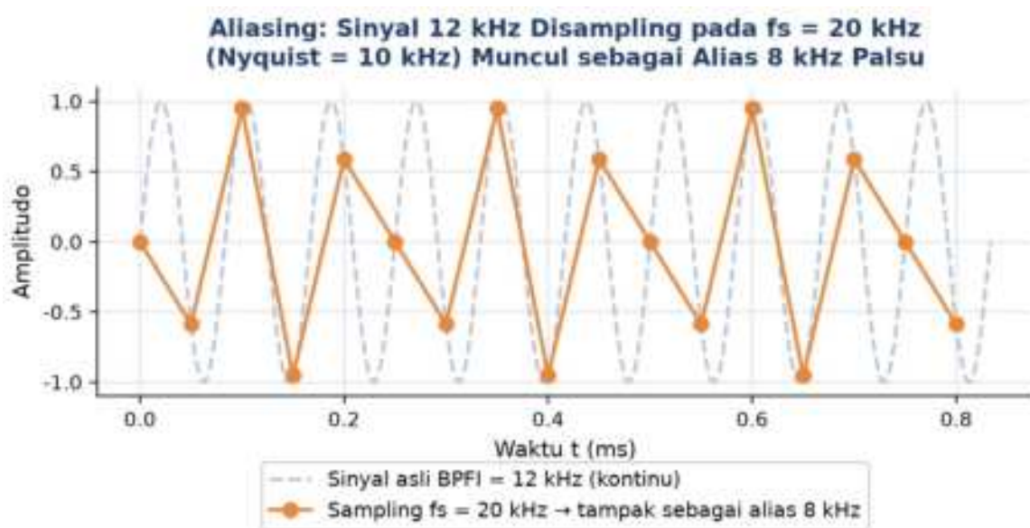
Gambar 5. Sinyal BPFI 12 kHz (kontinu, garis putus-putus) disampling pada f_s = 20 kHz (Nyquist = 10 kHz), menghasilkan titik-titik sample yang membentuk alias 8 kHz palsu.
