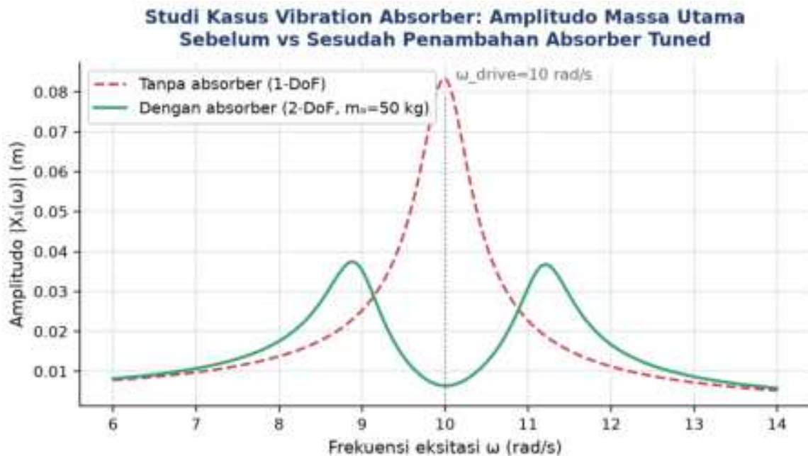
Gambar 6. Studi kasus vibration absorber: kurva amplitudo massa utama sebelum (garis putus merah, resonansi tunggal di \omega_{drive}=10 rad/s) dan sesudah penambahan absorber tuned (garis hijau, anti-resonansi di \omega_{drive} dengan dua puncak baru mengapit di 8,94 dan 11,18 rad/s).
