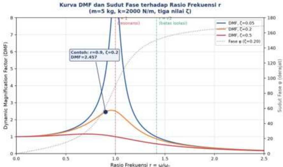
Gambar 4. Kurva DMF dan sudut fase terhadap rasio frekuensi r untuk tiga nilai \zeta , dengan marker resonansi ( r=1 ), batas isolasi ( r=\sqrt{2} ), dan contoh titik r=0,9 .
