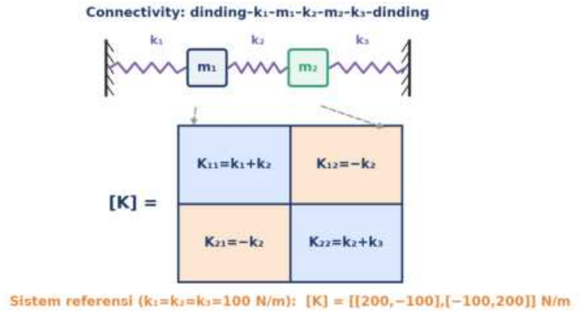
Gambar 4. Konstruksi matriks kekakuan [K] langsung dari connectivity sistem massa-pegas, tanpa perlu derivasi ulang Newton atau Lagrange.
