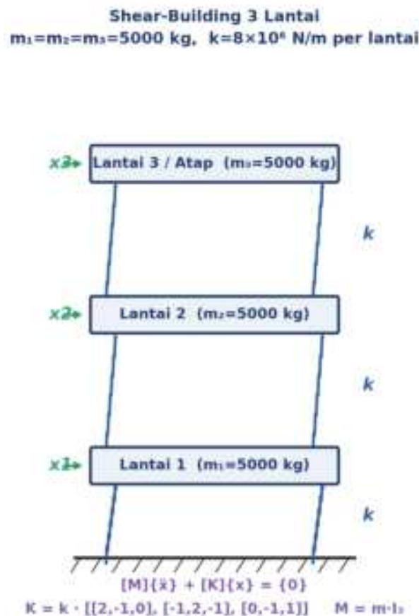
Gambar 2. Skematik shear-building 3 lantai: massa tiap lantai m=5000 kg, kekakuan antar-lantai k=8 \times 10^6 N/m, koordinat x_1, x_2, x_3 diukur dari posisi setimbang.
