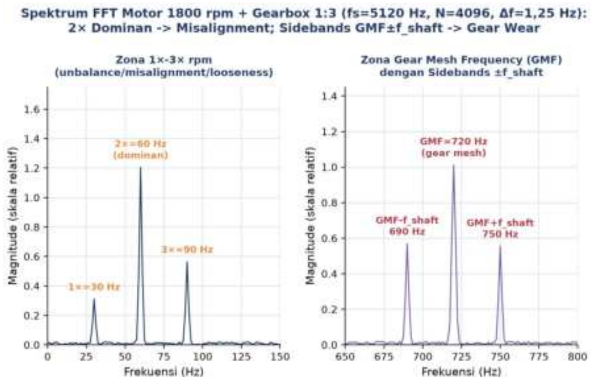
Gambar 7. Spektrum FFT motor 1800 rpm plus gearbox rasio 1:3: zona 1x-3x rpm (kiri) menunjukkan 2x dominan sebagai indikasi misalignment; zona gear mesh frequency (kanan) menunjukkan GMF 720 Hz dengan sidebands GMF plus-minus f_{\text{shaft}} sebagai indikasi gear wear.
