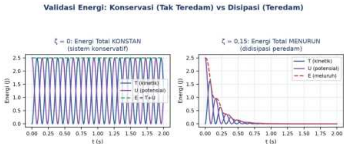
Gambar 7. Validasi energi: konservasi total (sistem tak teredam) versus disipasi monoton (sistem teredam) untuk parameter m=5 kg, k=2000 N/m.
