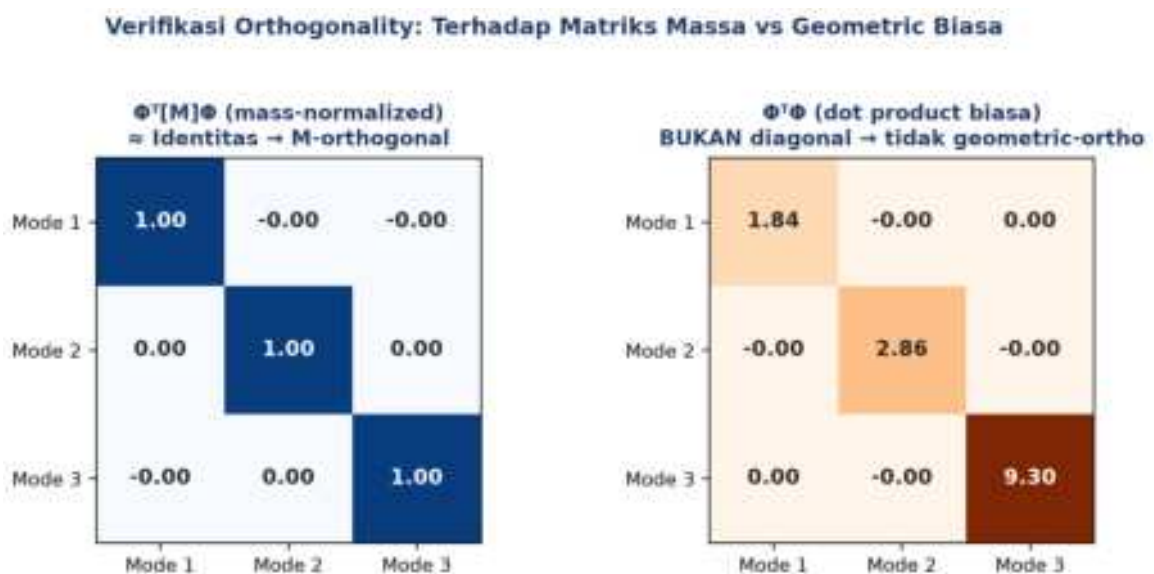
Gambar 5. Verifikasi orthogonality gedung 3 lantai: \Phi^T[M]\Phi (kiri) persis identitas, sedangkan \Phi^T\Phi (kanan, dot product geometris biasa) bukan matriks diagonal.
