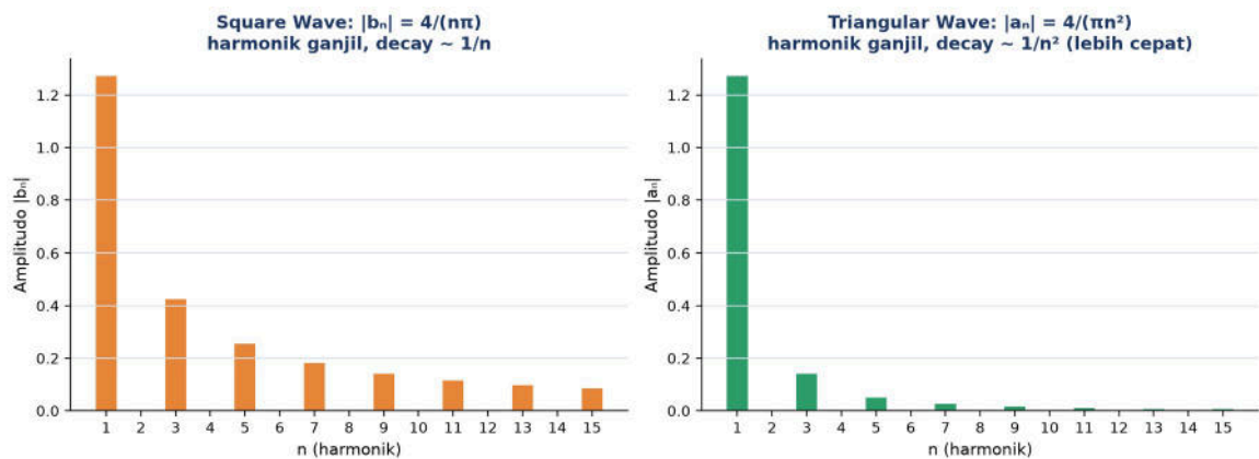
Gambar 2. Spektrum amplitudo square wave (decay \sim 1/n , harmonik ganjil) dibandingkan triangular wave (decay \sim 1/n^2 , harmonik ganjil), menunjukan laju peluruhan yang jauh lebih cepat pada sinyal yang lebih halus.
