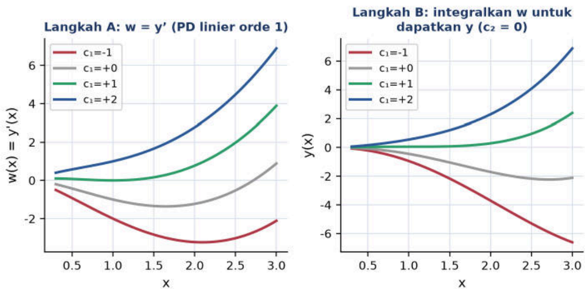
Gambar 6. Reduksi orde pada Contoh 4.7: panel kiri w(x) = y'(x) untuk empat nilai c_1 berbeda (PD linier orde satu hasil reduksi), panel kanan y(x) hasil integrasi ulang w dengan c_2 = 0 .
