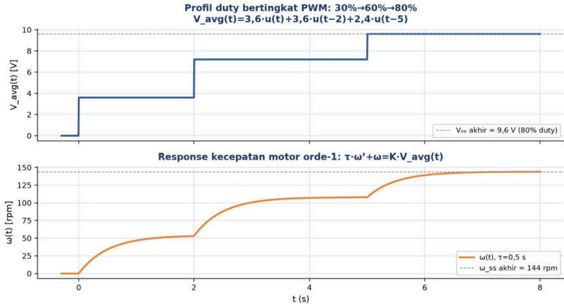
Gambar 7. Studi kasus PWM motor control : profil tegangan rata-rata V_g(t) hasil tiga step duty bertingkat (panel atas) dan response kecepatan motor \omega(t) orde- 1 dengan time constant \tau=0,5 detik (panel bawah).
