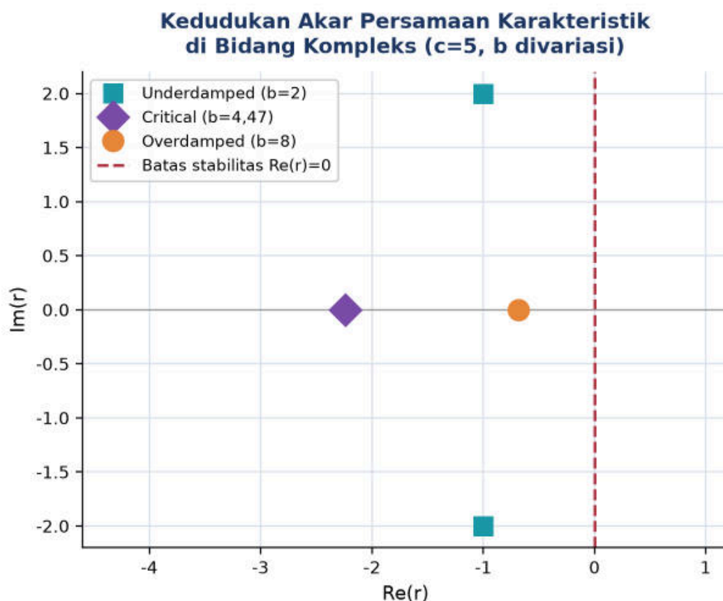
Gambar 3. Kedudukan akar persamaan karakteristik s^2 + bs + 5 = 0 di bidang kompleks untuk tiga nilai b yang sama dengan Gambar 2; garis putus-putus merah adalah batas stabilitas Re(r)=0 .
