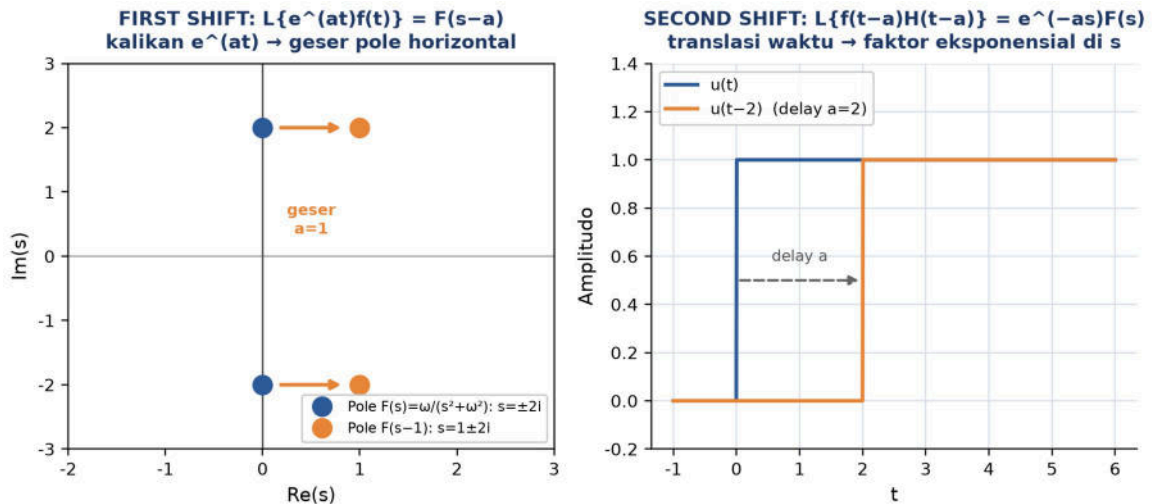
Gambar 3 | Ilustrasi First Shift Theorem (kiri, pole F(s) bergeser horizontal sejauh a saat dikalikan e^{at} ) dan Second Shift Theorem (kanan, fungsi step tertunda a dan dikalikan faktor e^{-as} di domain s ).
