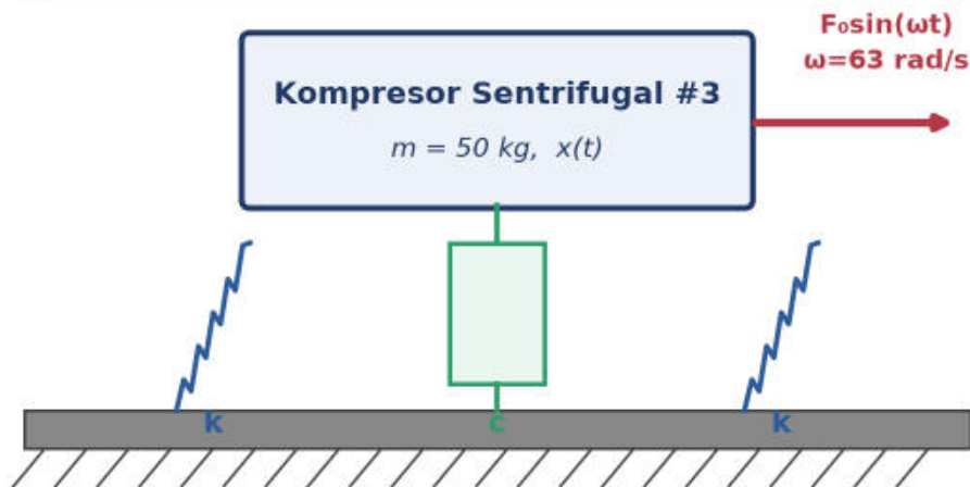
Gambar 6. Skema kompresor sentrifugal pada fondasi pegas- redaman mengalam near- resonansi: L(D)x = F_0 \sin(\omega t) dengan \omega operasi mendekati frekuensi natural fondasi \omega_n .
