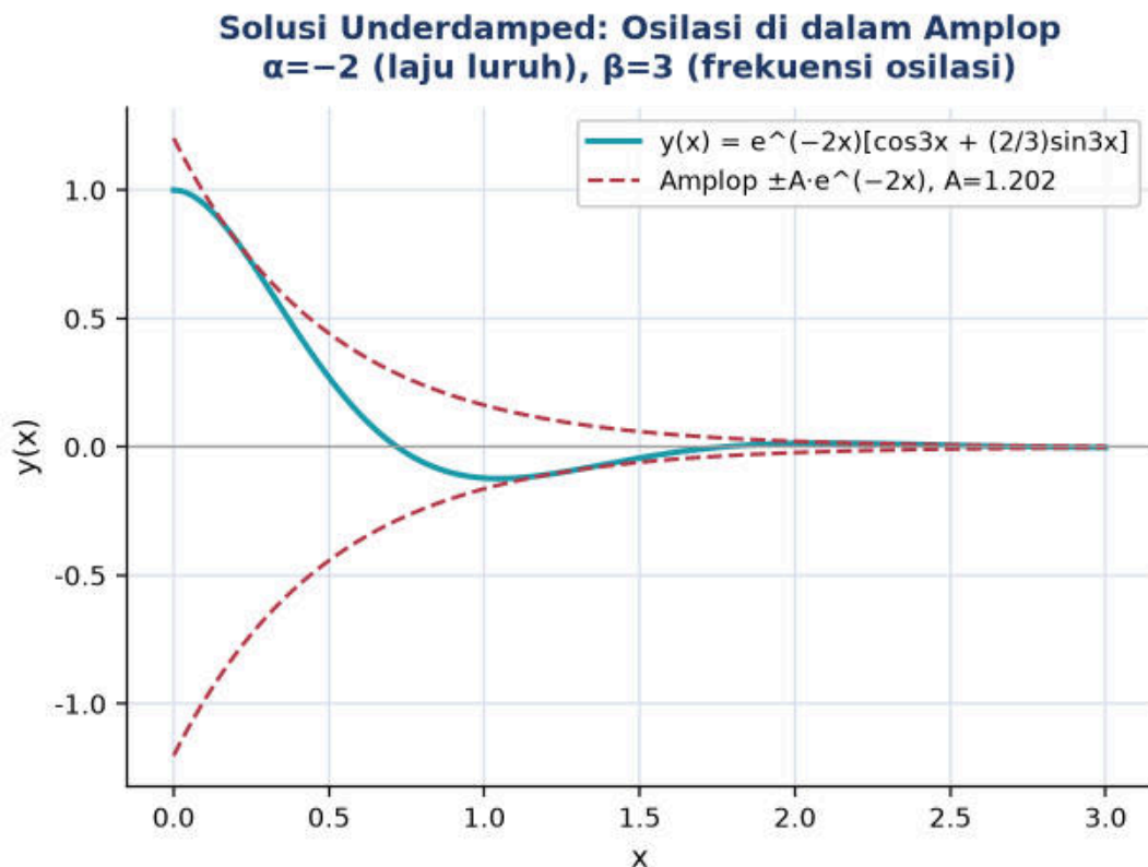
Gambar 5. Solusi underdamped PD y'' + 4y' + 13y = 0 , y(0)=1 , y'(0)=0 : kurva y(x)=e^{-2x}[\cos 3x + (2/3)\sin 3x] berosilasi di dalam amplop \pm Ae^{-2x} dengan A \approx 1,202 .
