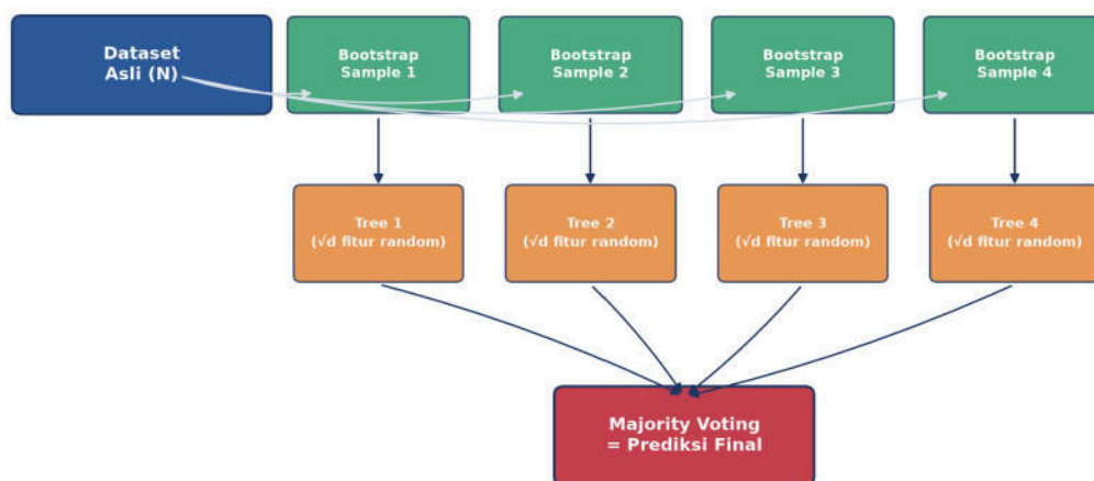
Gambar 2. Diagram Random Forest: data asli menghasilkan beberapa bootstrap sample, tiap sample melatih satu tree dengan subset fitur acak, prediksi akhir via majority voting.
