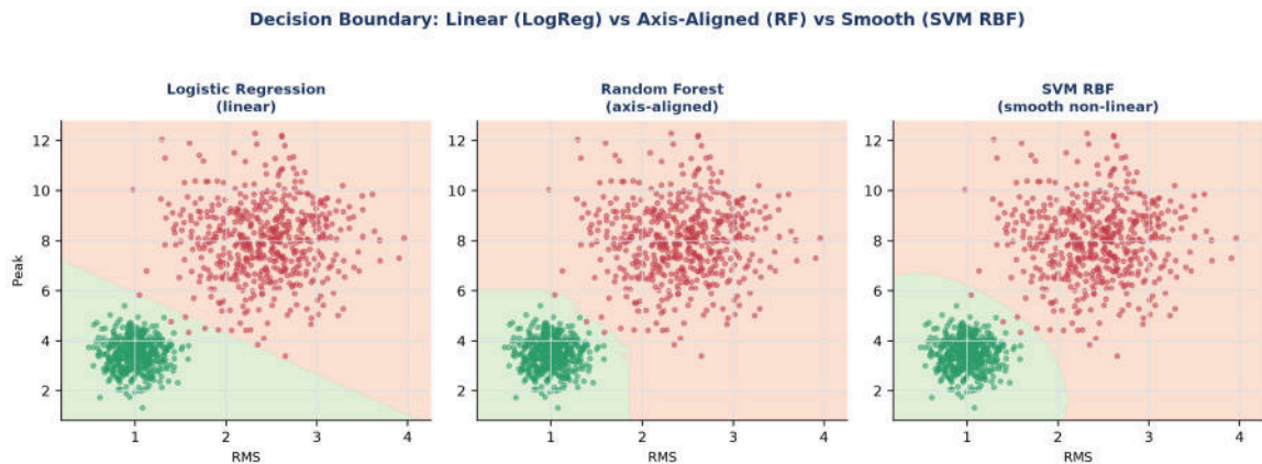
Gambar 3. Perbandingan decision boundary tiap algoritma pada data yang sama: linear (Logistic Regression), axis-aligned bertingkat (Random Forest), dan smooth non-linear (SVM RBF).
