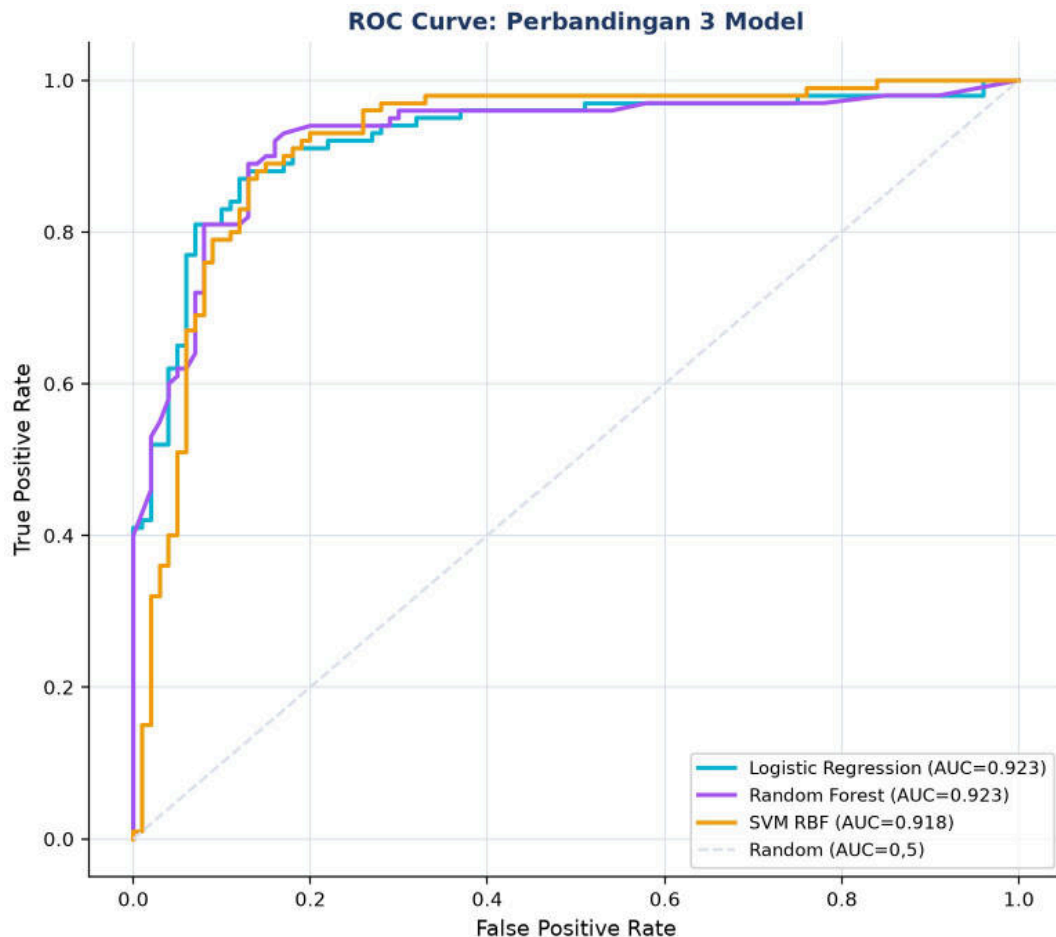
Gambar 4. Kurva ROC tiga model (Logistic Regression, Random Forest, SVM RBF) pada dataset dengan overlap kelas lebih realistis; AUC mengukur kemampuan model meranking sampel positif di atas negatif, independen dari threshold.
