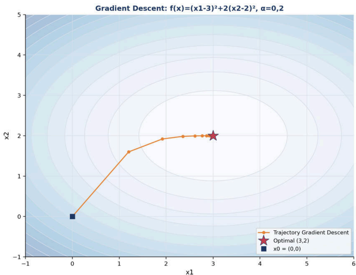
Gambar 2. Trajectory gradient descent pada kontur f(x) = (x_1 - 3)^2 + 2(x_2 - 2)^2 dari \mathbf{x}_0 = (0, 0) menuju optimal (3, 2) , \alpha = 0,2 .
