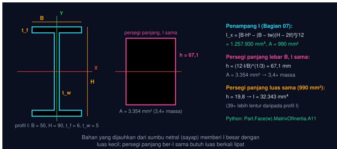
Gambar 6 — Penampang I versus persegi panjang dengan momen inersia sama. Profil I B = 50, H = 90, t_f = 6 , t_w = 5 memiliki I_x = 1.257.930 \text{ mm}^4 dengan luas 990 \text{ mm}^2 ; persegi panjang selebar B yang sama kakunya harus setinggi 67,1 mm dengan luas 3.354 \text{ mm}^2 , 3,4 kali massa.
