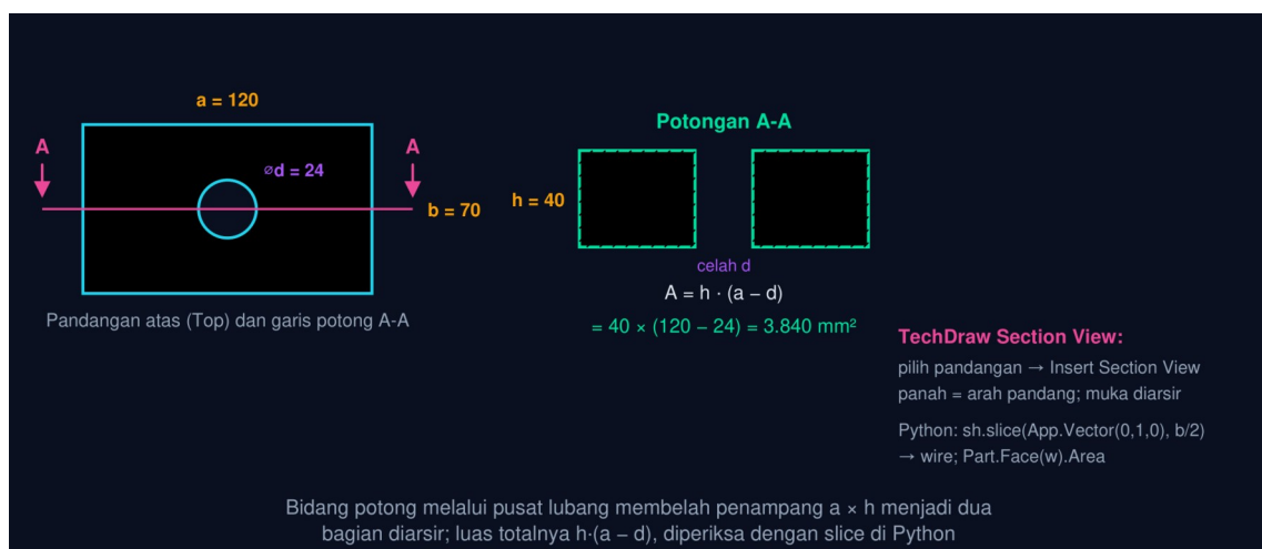
Gambar 5 — Section View A-A balok berlubang dan luas penampang potongan. Balok 120 \times 70 \times 40 berlubang \varnothing 24 dipotong bidang y = b/2 melalui pusat lubang: penampang 120 \times 40 terbelah celah selebar d, luas totalnya h \cdot (a - d) = 3.840 \text{ mm}^2 .
