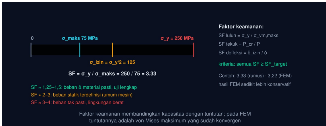
Gambar 4 — Skala tegangan, tegangan izin, dan faktor keamanan terhadap luluh. Kantilever contoh: \sigma_{maks} = 75 MPa terhadap \sigma_y = 250 MPa memberi SF = 3,33; dengan SF target 2, tegangan izin \sigma_y/2 = 125 MPa masih jauh di atas tegangan kerja.
