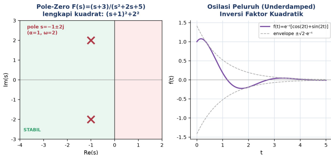
Gambar 4. Pole kompleks konjugat s=-1 plus-minus 2j hasil melengkapi kuadrat (s+1)^2+2^2 (kiri) dan respons underdamped f(t)=e^{-t}[\cos(2t)+\sin(2t)] dengan envelope peluruh (kanan).
